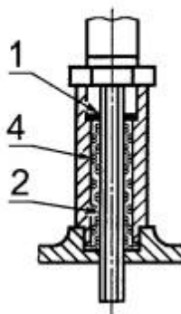
Рисунок 3 - Иллюстрация места ввода корешка и разделки (развода жил)
