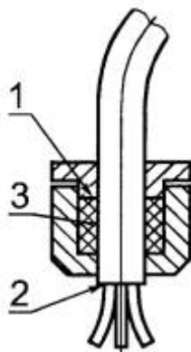
а) Кабельный ввод
