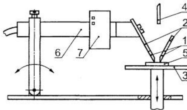
Рисунок 3 - Образец испытательного устройства
