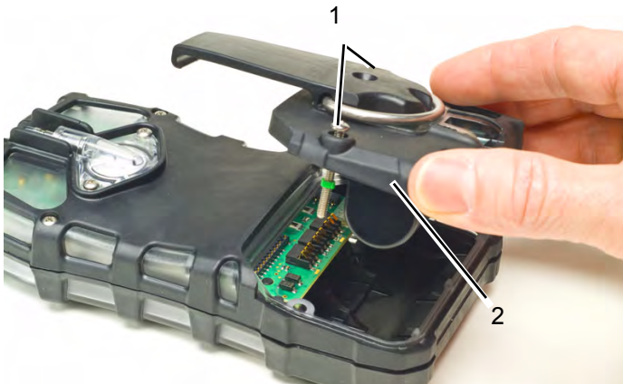
Рис. 12 Замена батареи
