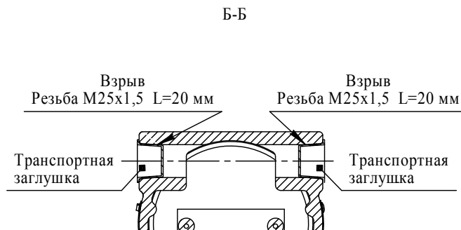
Рисунок Е.1 - Чертеж средств взрывозащиты газоанализаторов ДАК-СО 2 -126, ДАК-СН 4 -129, ДАК-СН 4 -137, ДАК-ΣСН-138, ДАК-ΣСН-139
