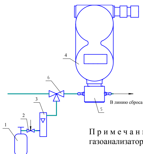
Рисунок 3.1 – Схема для проведения проверки (корректировки) нулевых показаний и чувствительности газоанализаторов
