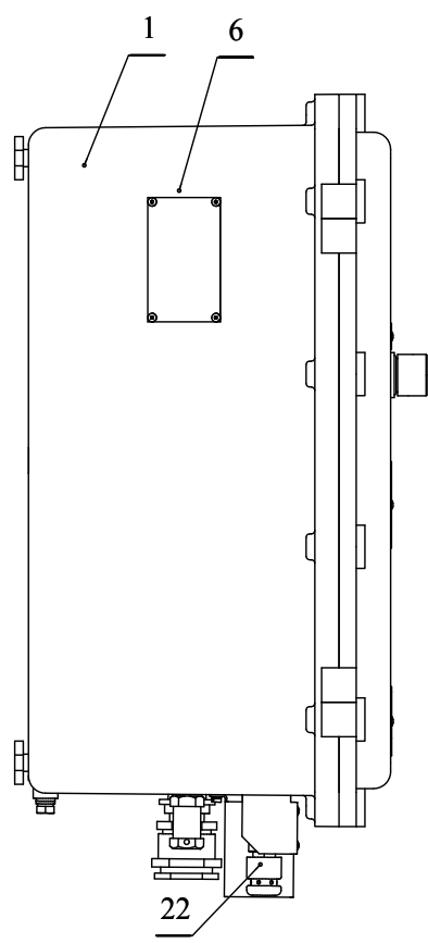
Внешний вид газоанализатора со снятой крышкой (2)
