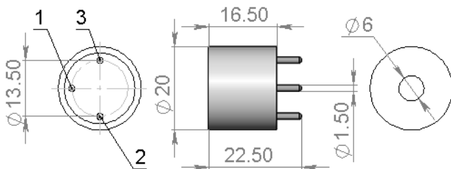
Рис.1 Размеры сенсора и схема расположения выводов 1 - индикаторный электрод 2 - вспомогательный электрод 3 - электрод сравнения
