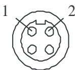
Рисунок 7.5 Вид со стороны пайки
