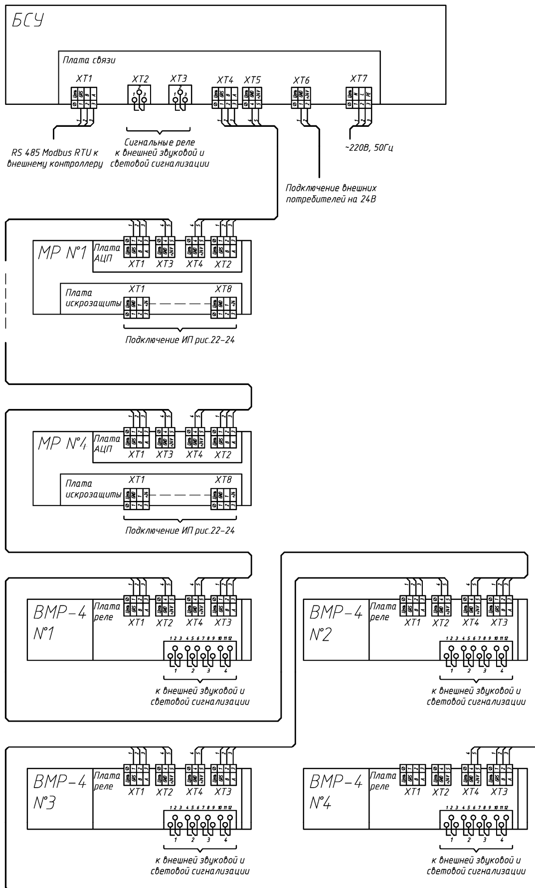
Рис.В.20. Схема подключения блоков системы. Вариант 6.
