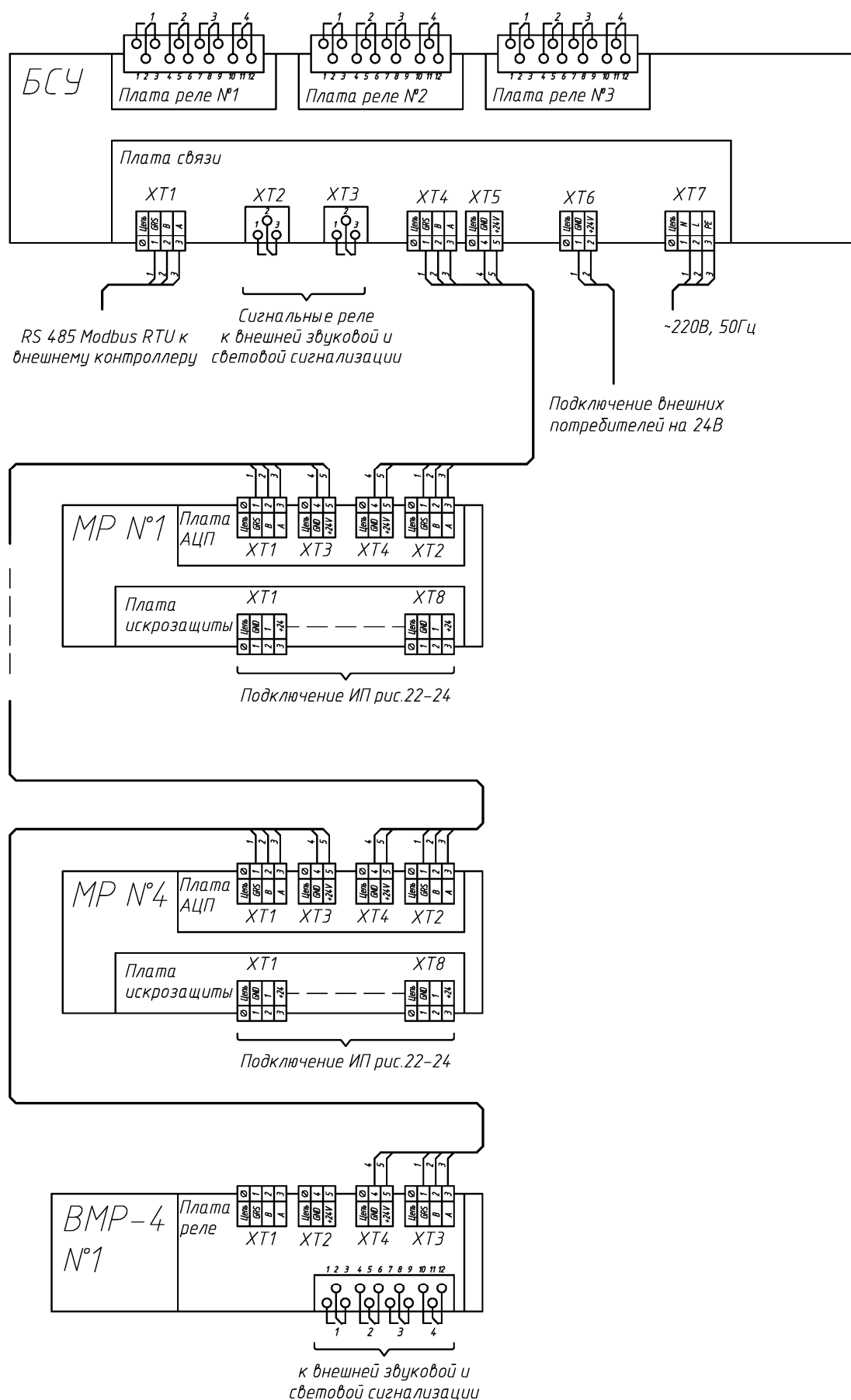
Рис.В.16. Схема подключения блоков системы. Вариант 2.
