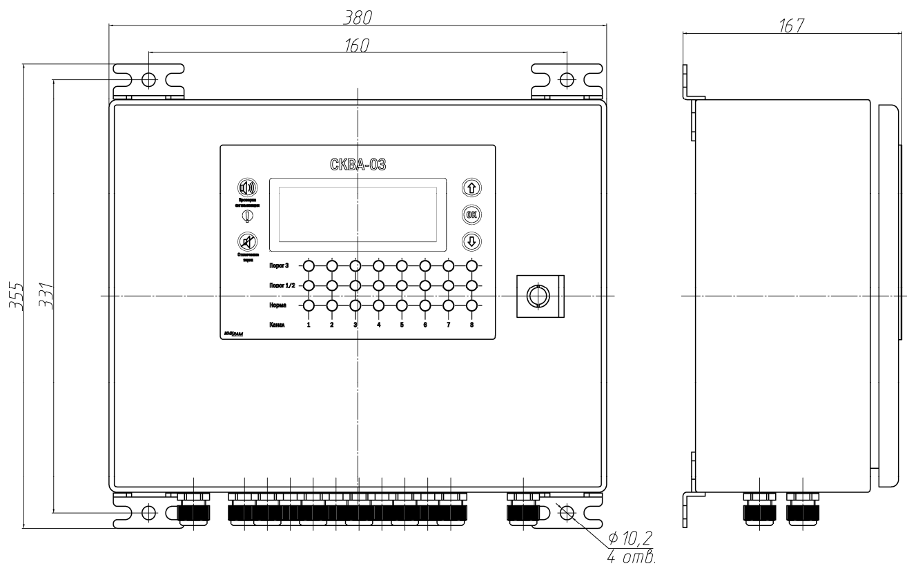
Рис.В.1. БСУ-Ех и БСУ-0. Общий вид, габаритные и присоединительные размеры.
