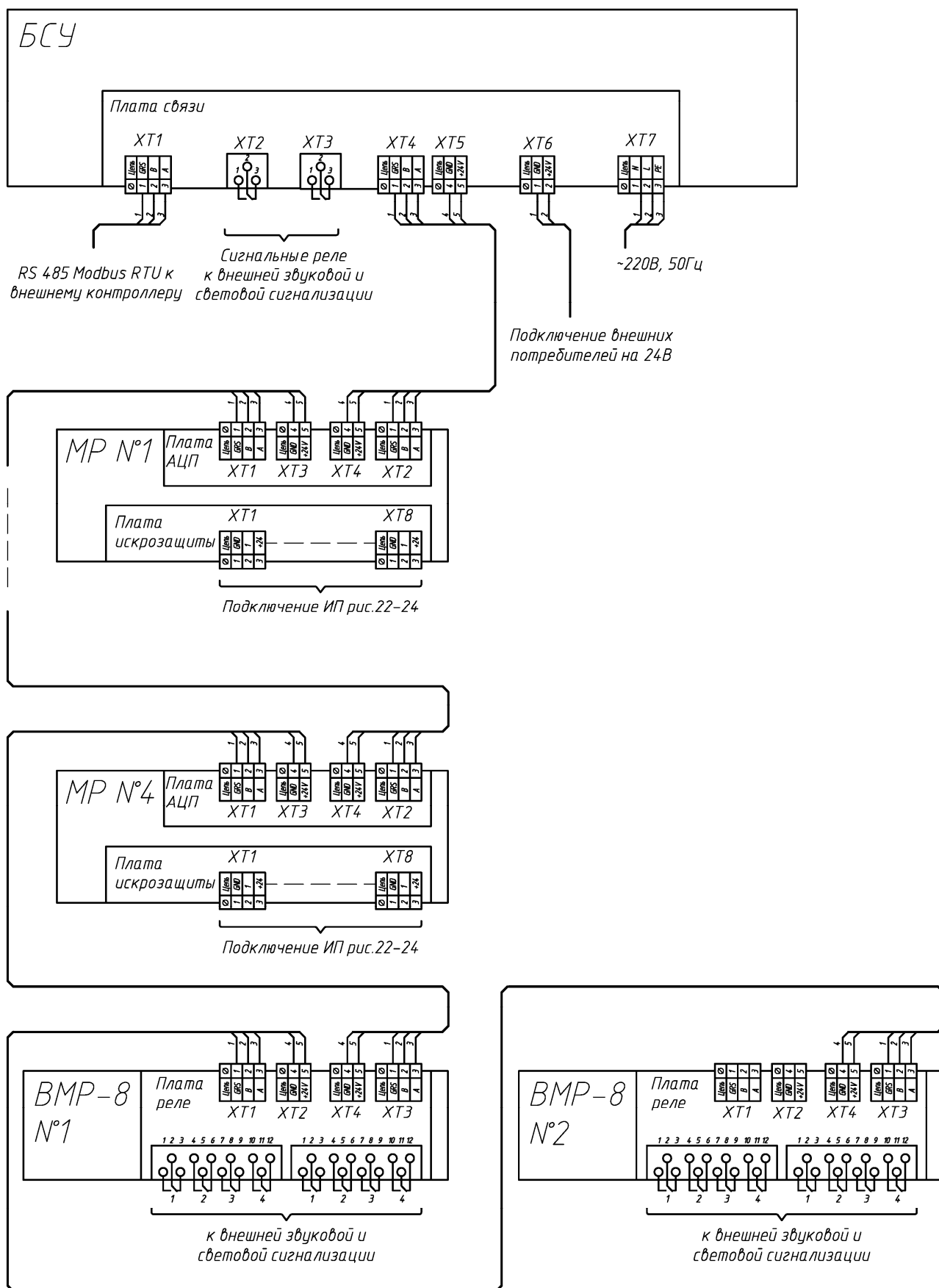
Рис.В.21. Схема подключения блоков системы. Вариант 7.
