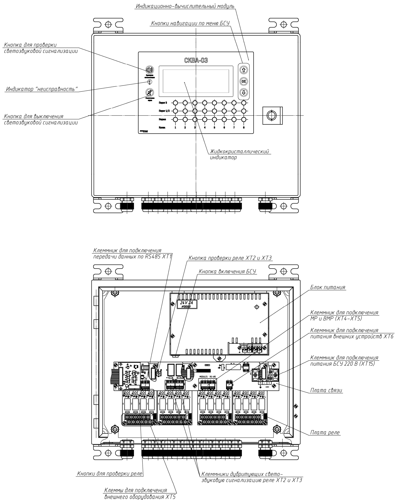
Рис.В.2. БСУ-Ех. Состав.
