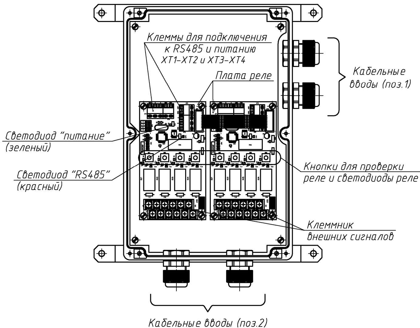
Рис.В.13. BMP8-Ex и BMP8-0. Состав.
