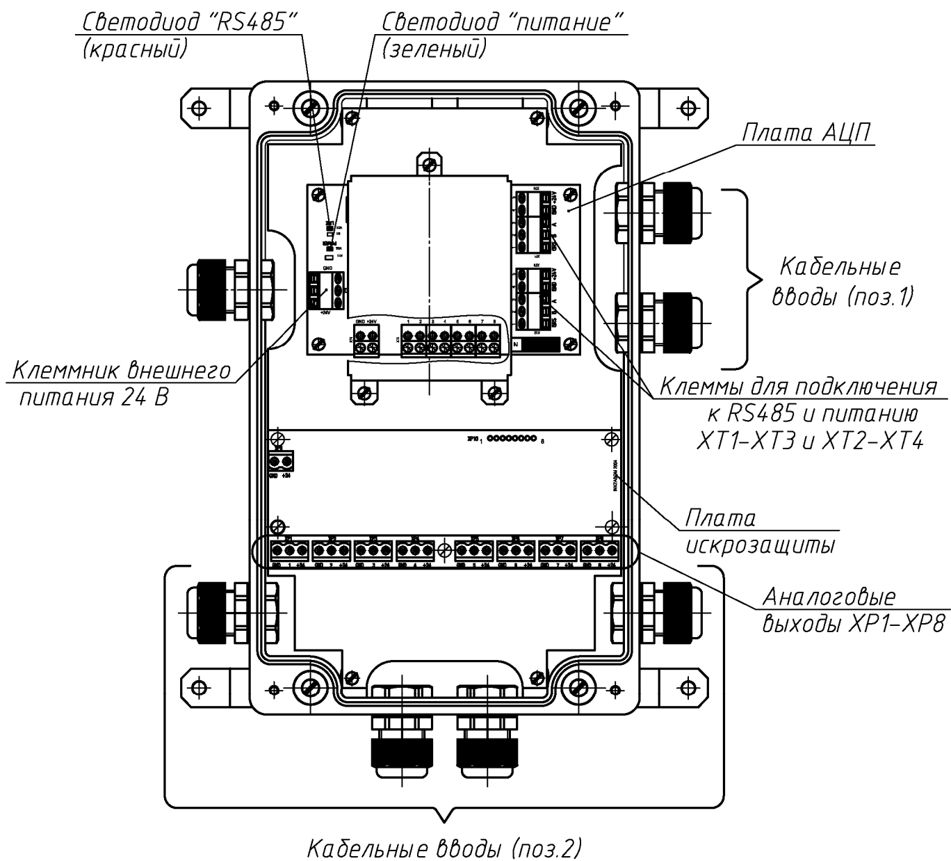
Рис.В.11. MP8-0-MK. Состав.
