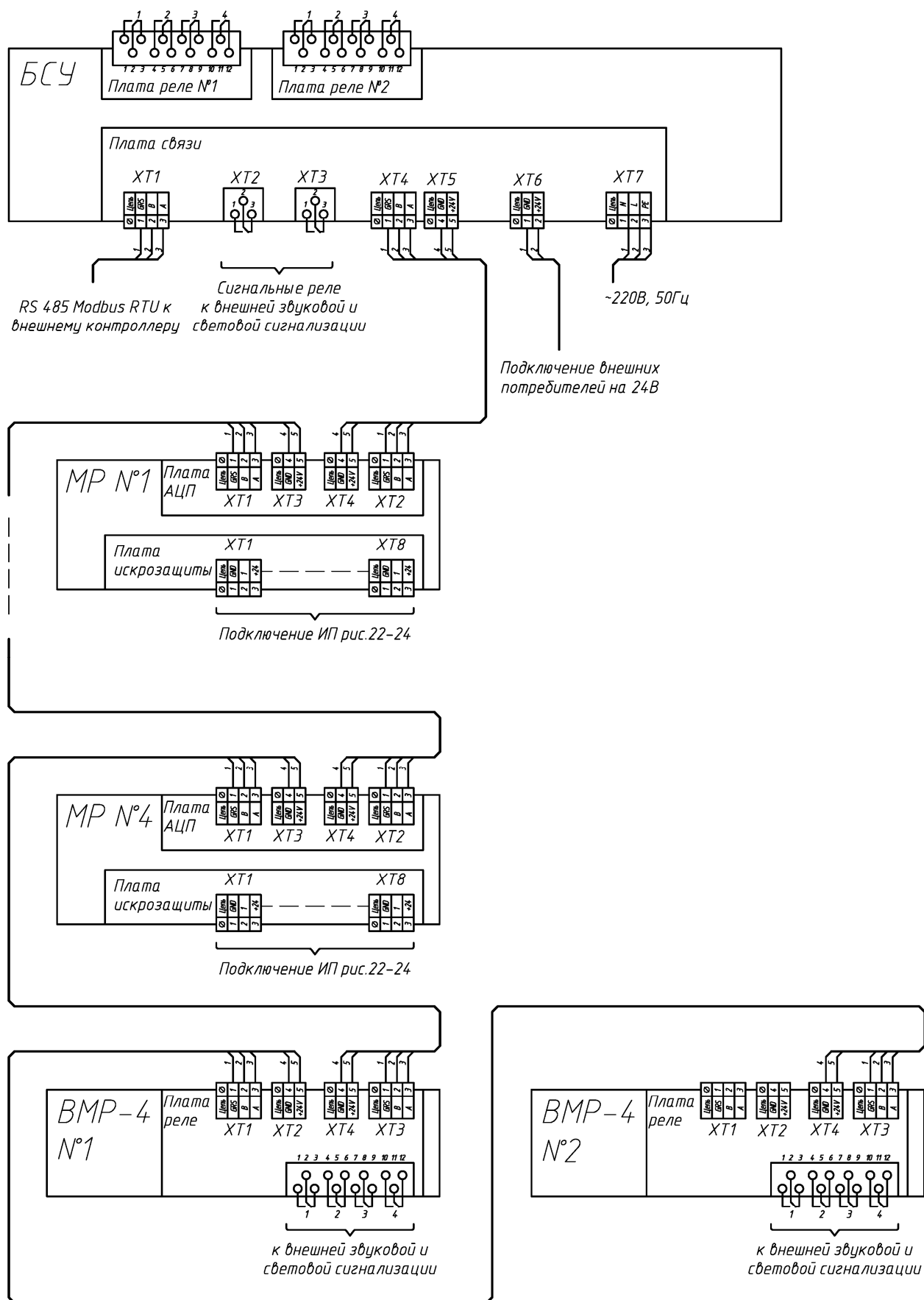
Рис.В.17. Схема подключения блоков системы. Вариант 3.
