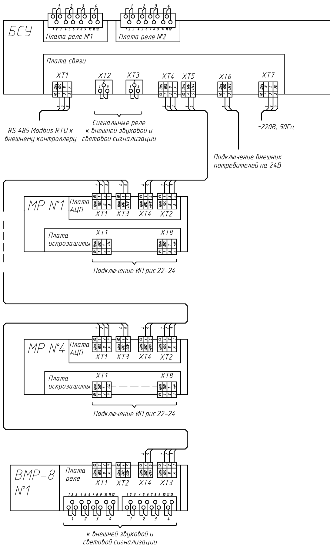
Рис.В.18. Схема подключения блоков системы. Вариант 4.
