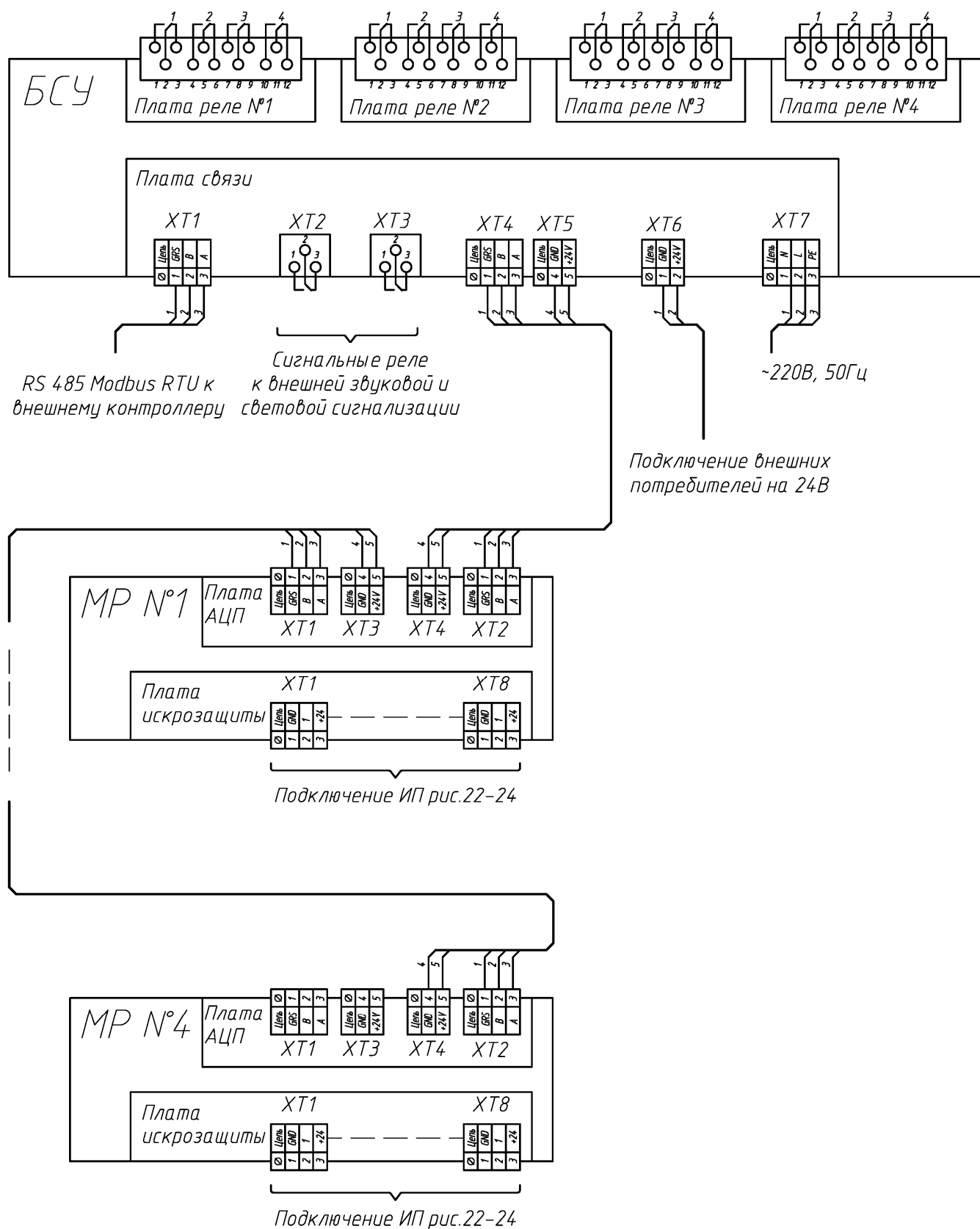
Рис.В.15. Схема подключения блоков системы. Вариант 1.
