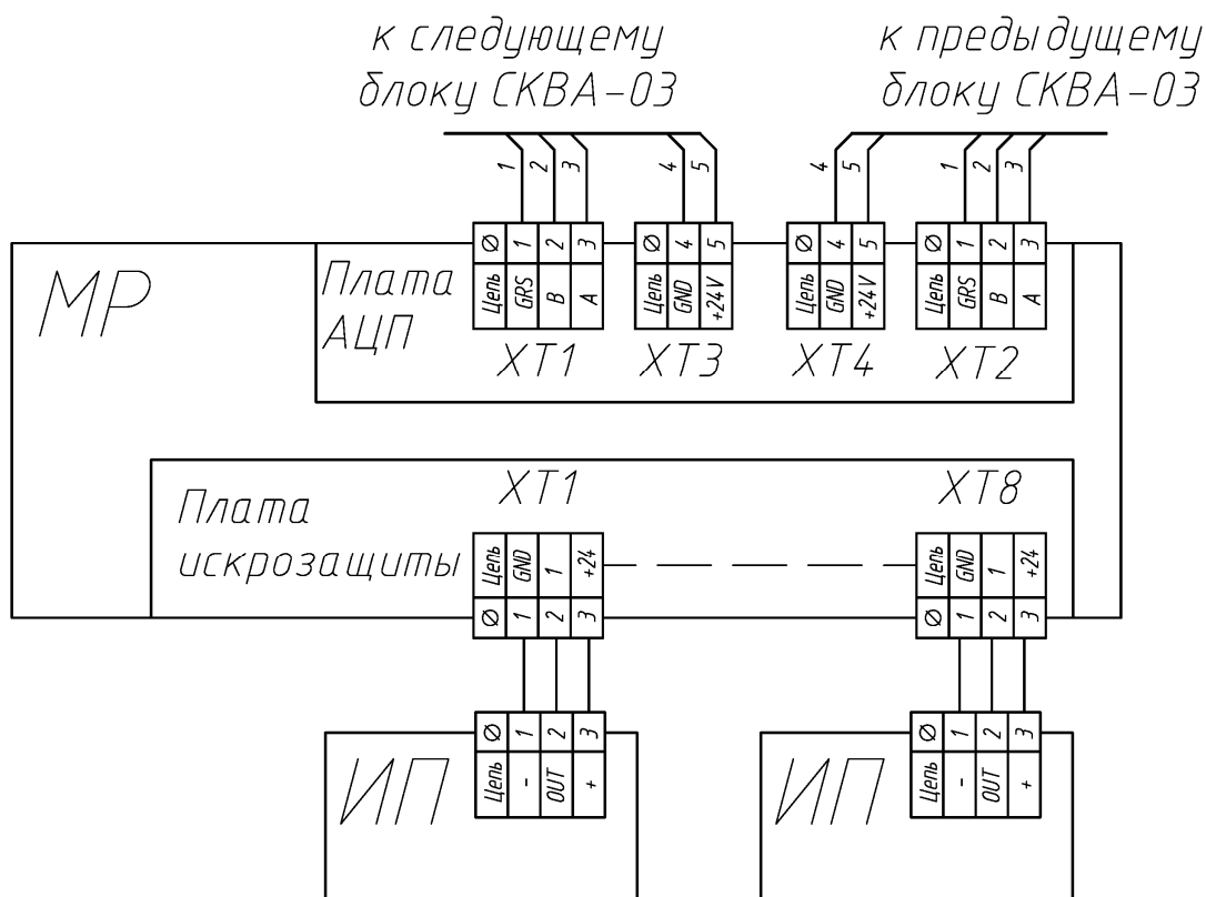
Рис.В.23. Схема подключения преобразователей измерительных серии А300.
