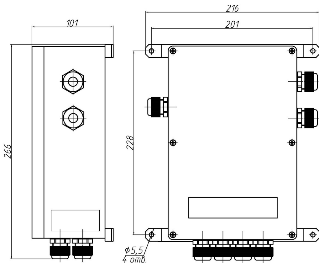
Рис.В.4. MP8-Ex. Общий вид, габаритные и присоединительные размеры.
