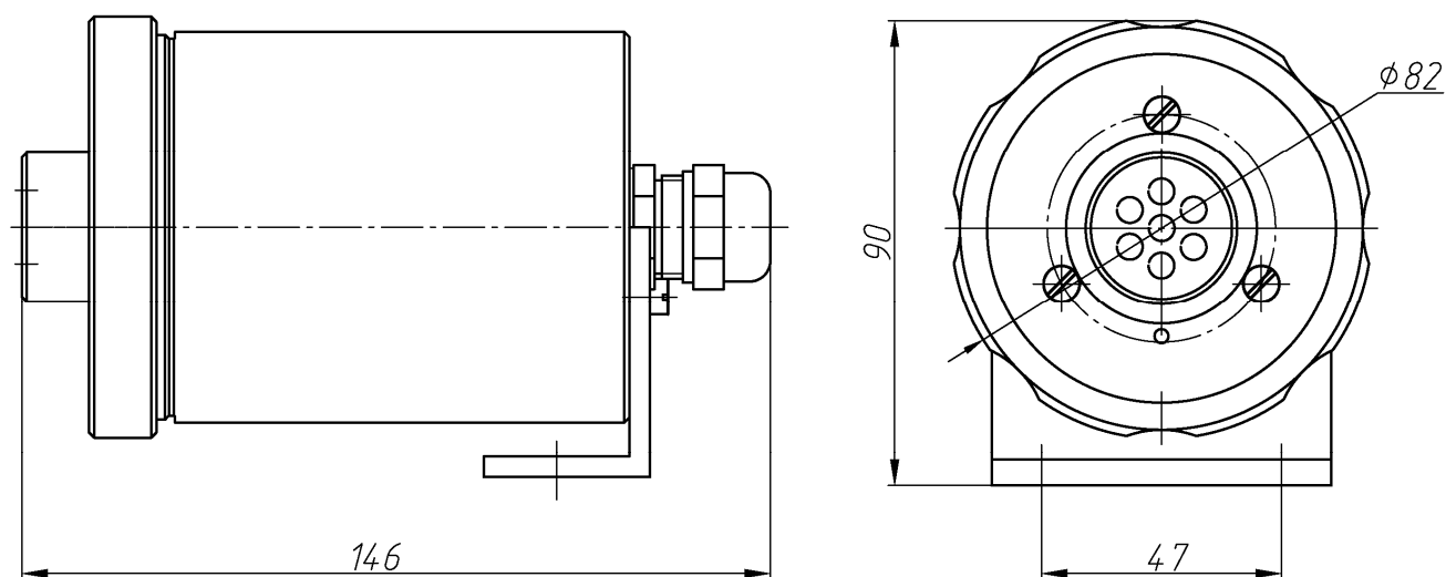
Рис. В.27. ИП серии В3ХХ и С3ХХ. Общий вид, габаритные и присоединительные размеры.
