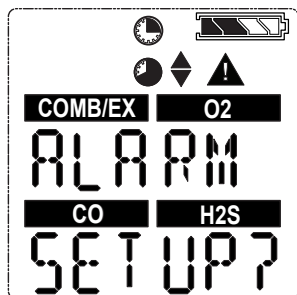
Рис. 6 Настройка сигнализации
