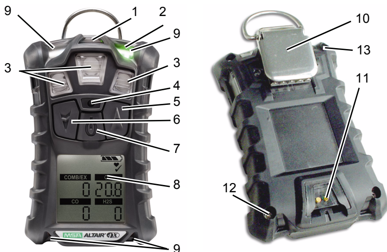
Рис. 1 Обзор прибора
