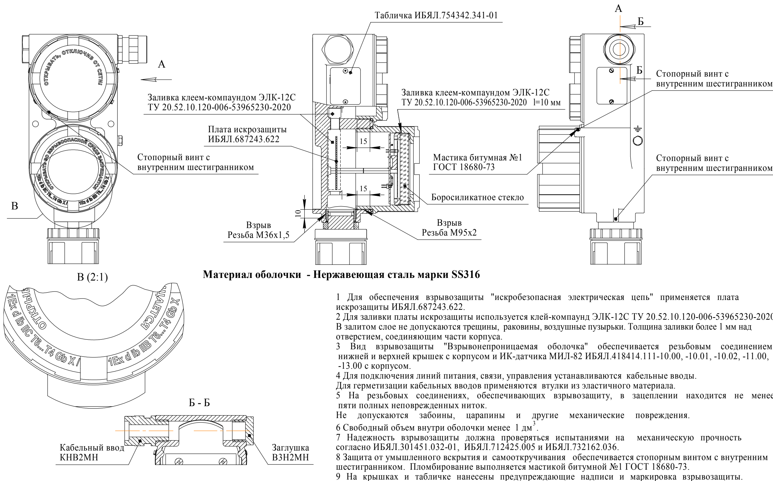
Рисунок Е.3 - Чертеж средств взрывозащиты газоанализаторов ДАК-СО 2 -131, ДАК-СН 4 -132, ДАК-ΣСН-133 (материал оболочки - нержавеющая сталь)
