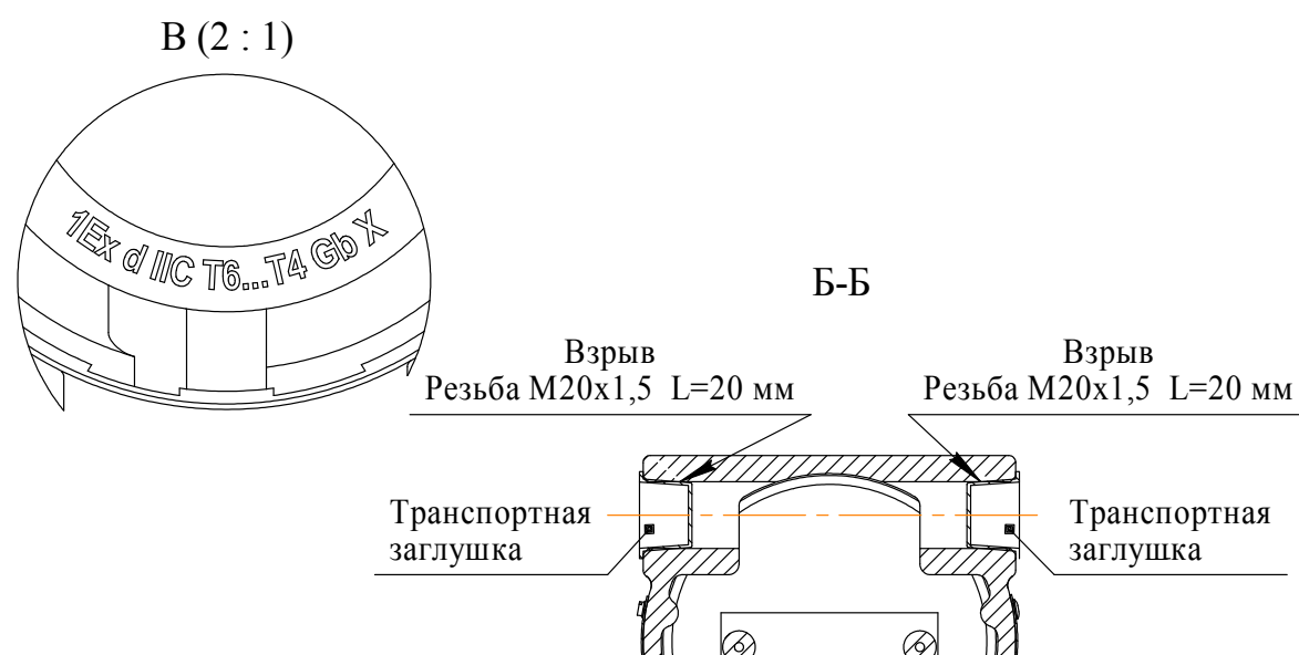
Рисунок Е.2 - Чертеж средств взрывозащиты газоанализаторов ДАК-СО 2 -126, ДАК-СН 4 -129, ДАК-СН 4 -137, ДАК-ΣСН-138, ДАК-ΣСН-139
