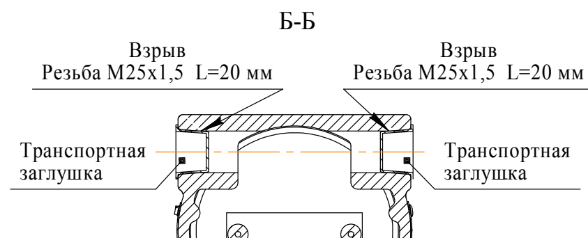
Рисунок Е.1 - Чертеж средств взрывозащиты газоанализаторов ДАК-СО 2 -126, ДАК-СН 4 -129, ДАК-СН 4 -137, ДАК-ΣСН-138, ДАК-ΣСН-139
