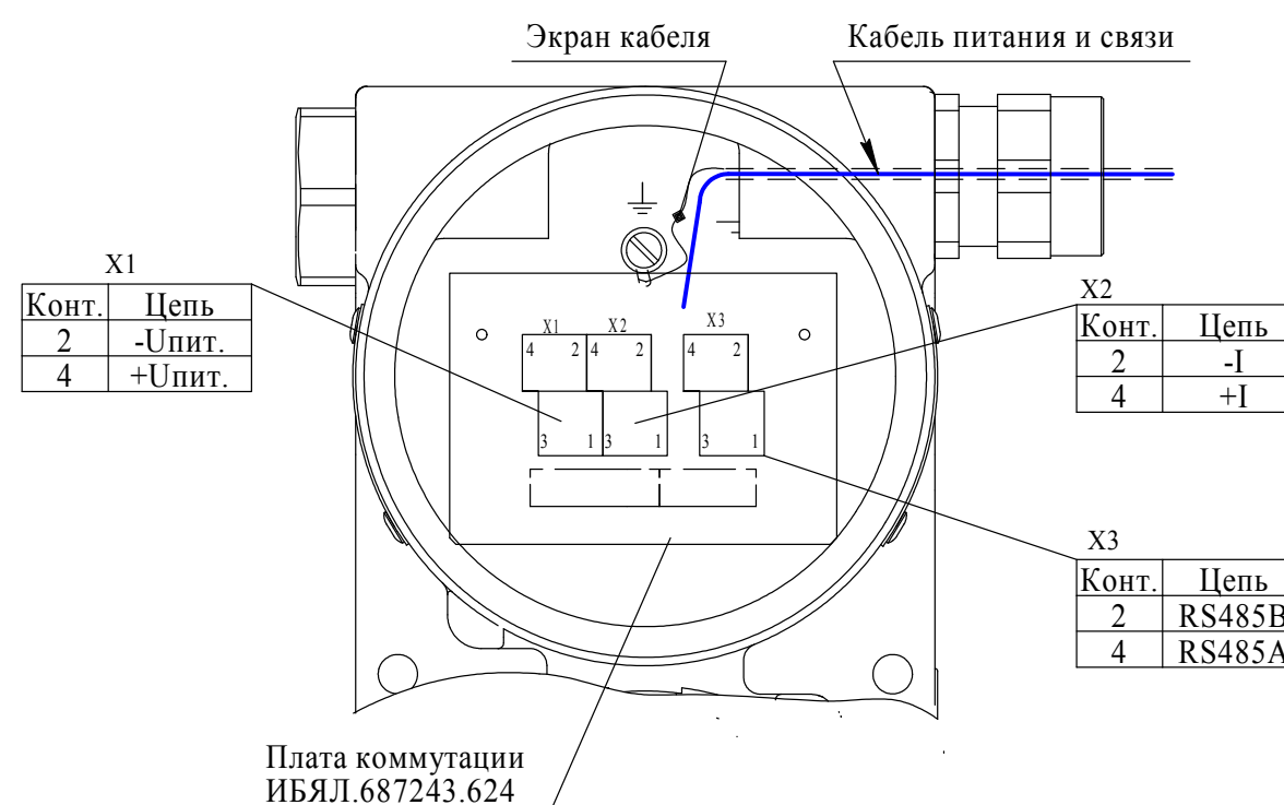
Рисунок платы коммутации газоанализаторов ДАК-СО 2 -131, ДАК-СН 4 -132, ДАК-ΣСН-133 с подходящими кабелями питания, связи
