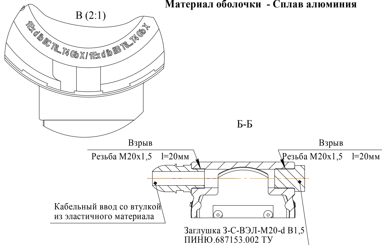
Рисунок Е.4 - Чертеж средств взрывозащиты газоанализаторов ДАК-СО 2 -131, ДАК-СН 4 -132, ДАК-ΣСН-133 (материал оболочки - сплав алюминия)
