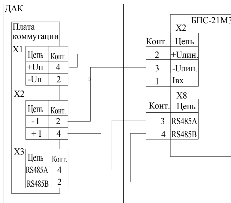
Рисунок Л.4 - Подключение газоанализаторов к БПС-21М3 ИБЯЛ.411111.047/-01/-02/-03/-04
