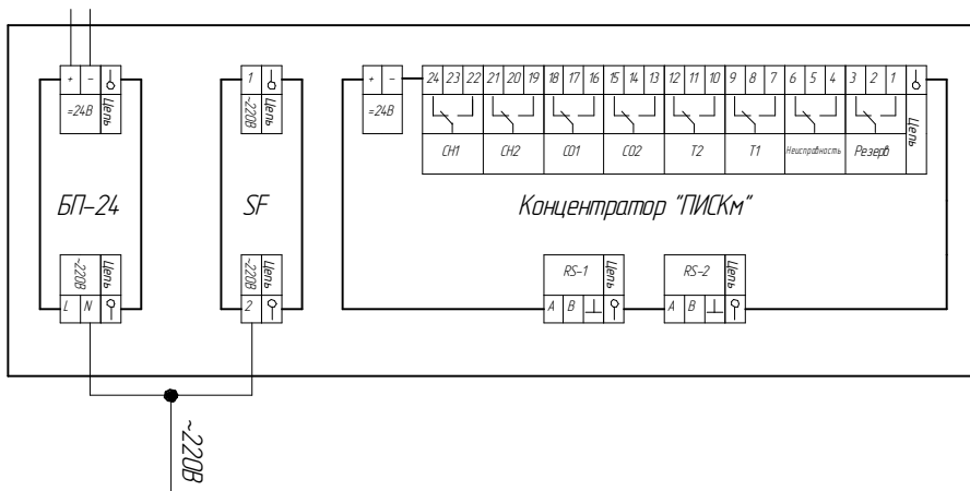
Рис. 2б. Описание дискретных выводов ПИСКм.152, ПИСКм.202, ПИСКм.302, ПИСКм.402 с отключённым питанием
