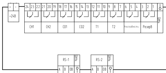
Рис. 2а. Описание дискретных выводов ПИСКм.100 с отключенным питанием
