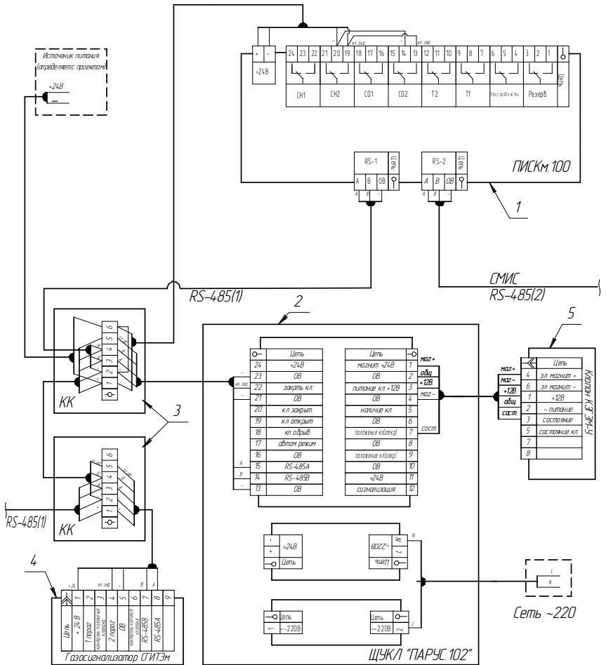
Рис. 5а. Пример схемы подключения системы контроля загазованности со смешанным автоматическим/автоматизированным управлением исполнительными устройствами, на основе ПИСКм.100, газосигнализаторов СГИТЭм, щита управления клапаном «ПАРУС.102» и блока управления импульсным клапаном «БУИК.301»
