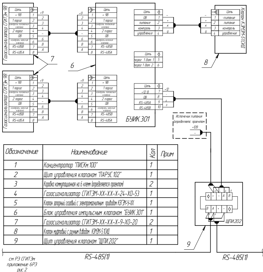
Окончание рис. 5. Пример схемы подключения системы контроля загазованности со смешанным автоматическим/автоматизированным управлением исполнительными устройствами, на основе изделия, газосигнализаторов СГИТЭМ, щита управления клапаном «ПАРУС.102» и блока управления импульсным клапаном БУИК.301»
