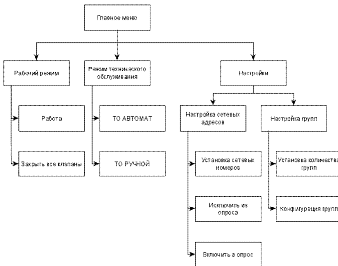
Рис. 1. Схема меню.
