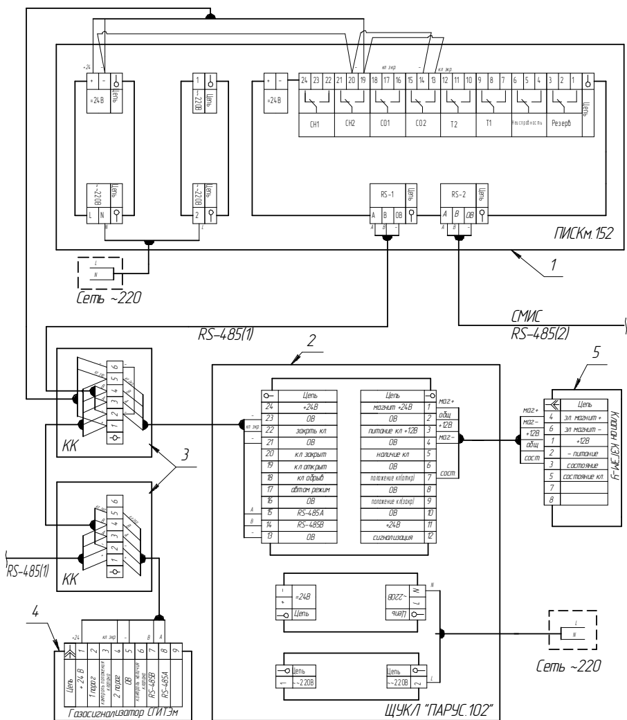
Рис. 5б. Пример схемы подключения системы контроля загазованности со смешанным автоматическим/автоматизированным управлением исполнительными устройствами, на основе ПИСКм.ХХ2, газосигнализаторов СГИТЭМ, щита управления клапаном «ПАРУС.102» и блока управления импульсным клапаном «БУИКС.301»
