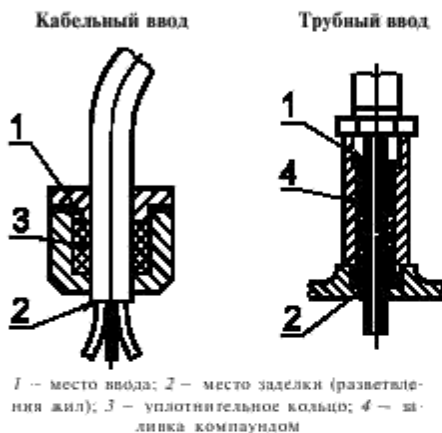
Рисунок 2 — Место ввода и заделки кабеля (разветвления жил)
