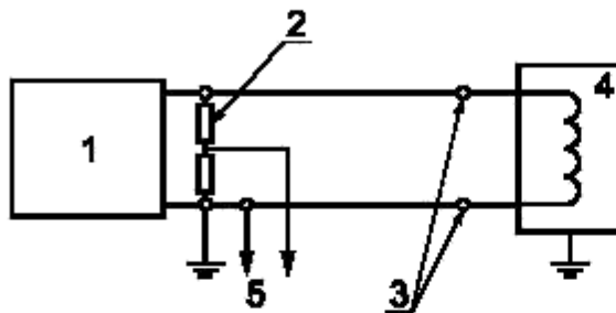
1 - генератор импульсов; 2 - делитель напряжения; 3 - соединительные контактные зажимы; 4 - испытуемое балластное устройство; 5 - контактные зажимы для присоединения электрического осциллографа
