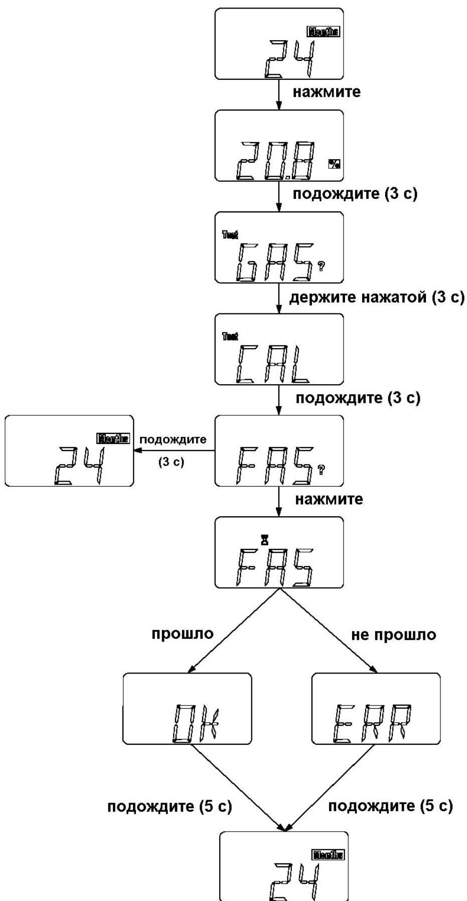
Рис. 9 Калибровка - Кислород
