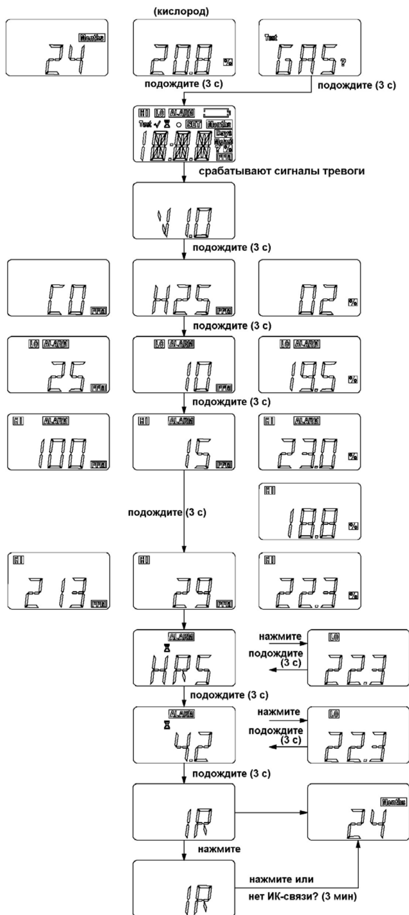
Рис.5 Считывание данных сигнализатора
