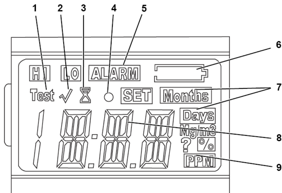
Рис. 2. Дисплей сигнализатора
