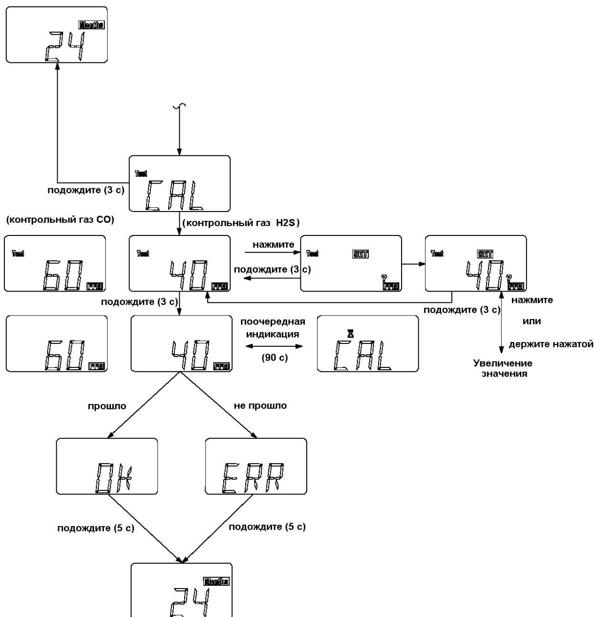
Рис. 8 Калибровка - Токсичные газы ( продолжение)
