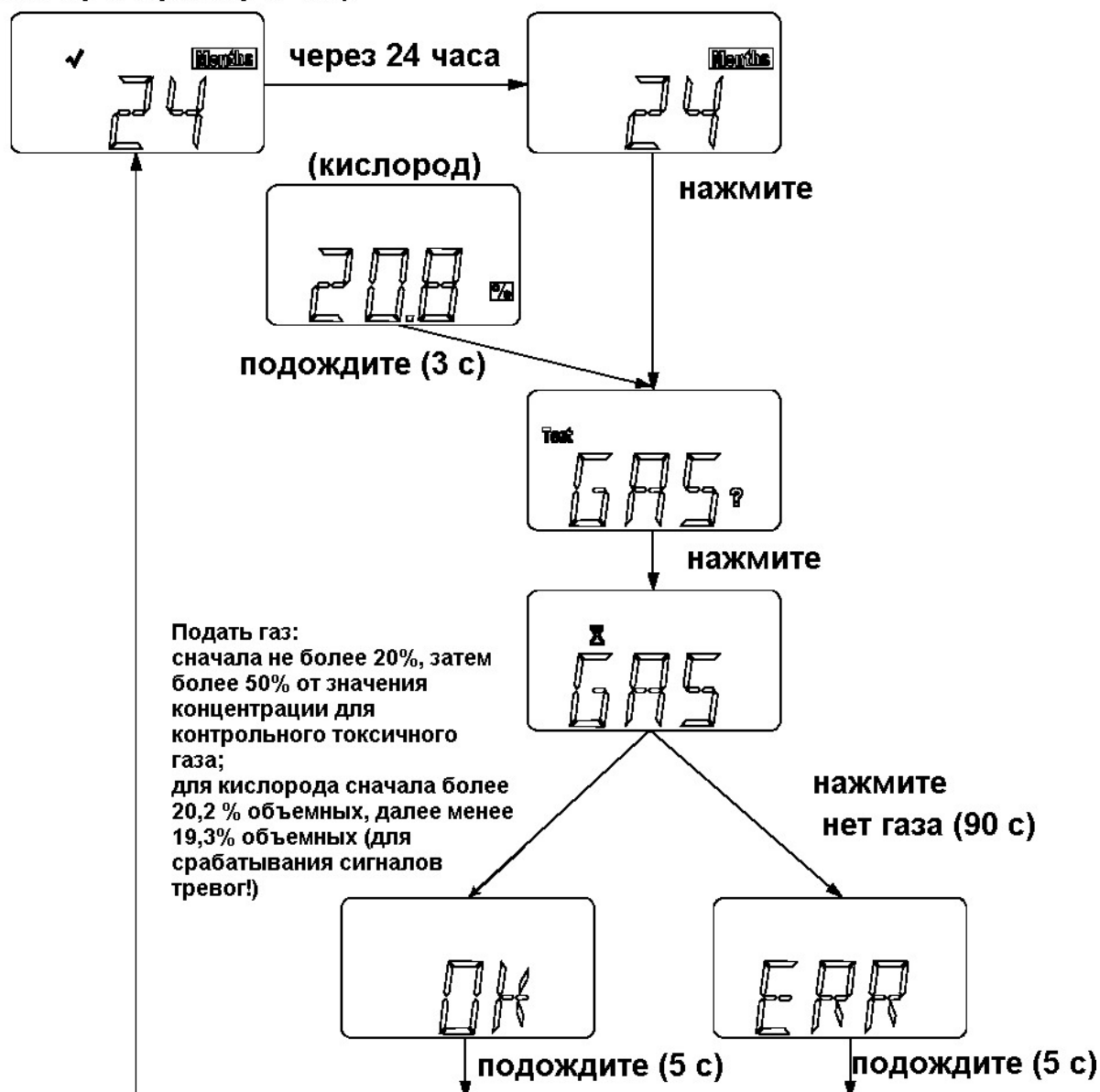
Рис. 6 Проведение проверки работоспособности
