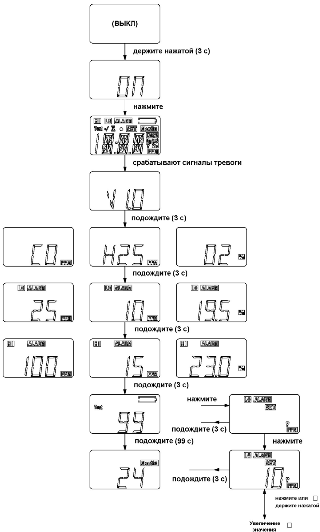
Рис. 4 Запуск сигнализатора
