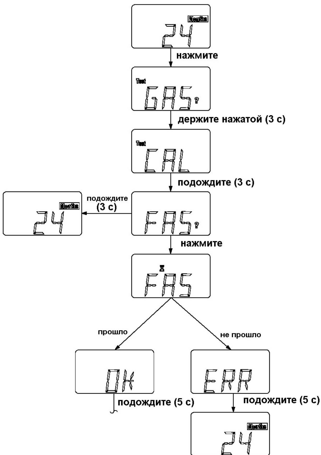
Рис. 7 Калибровка – Токсичные газы
