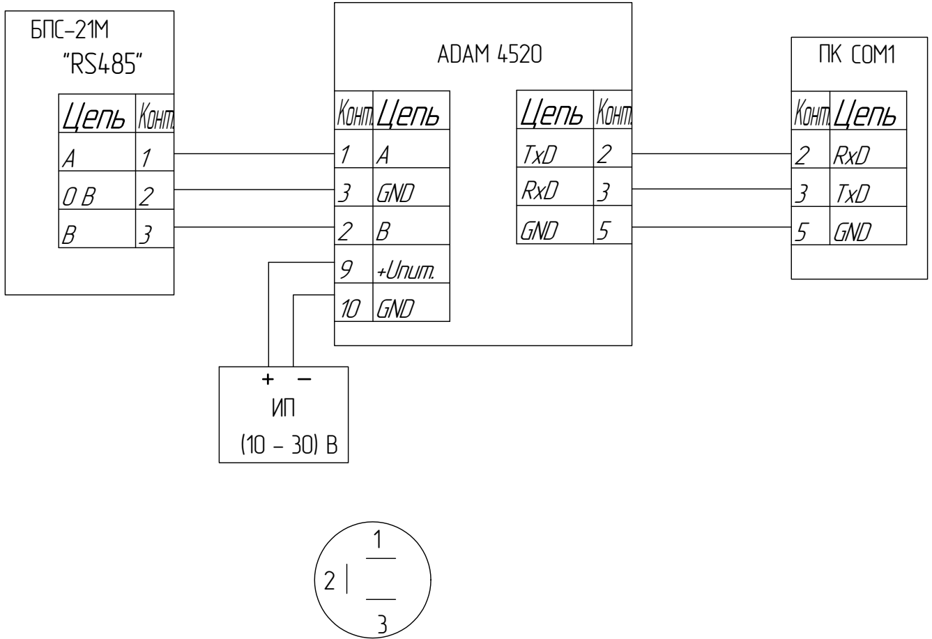
Рисунок 2.1 – Схема подключения блоков к ПК через адаптер интерфейса
