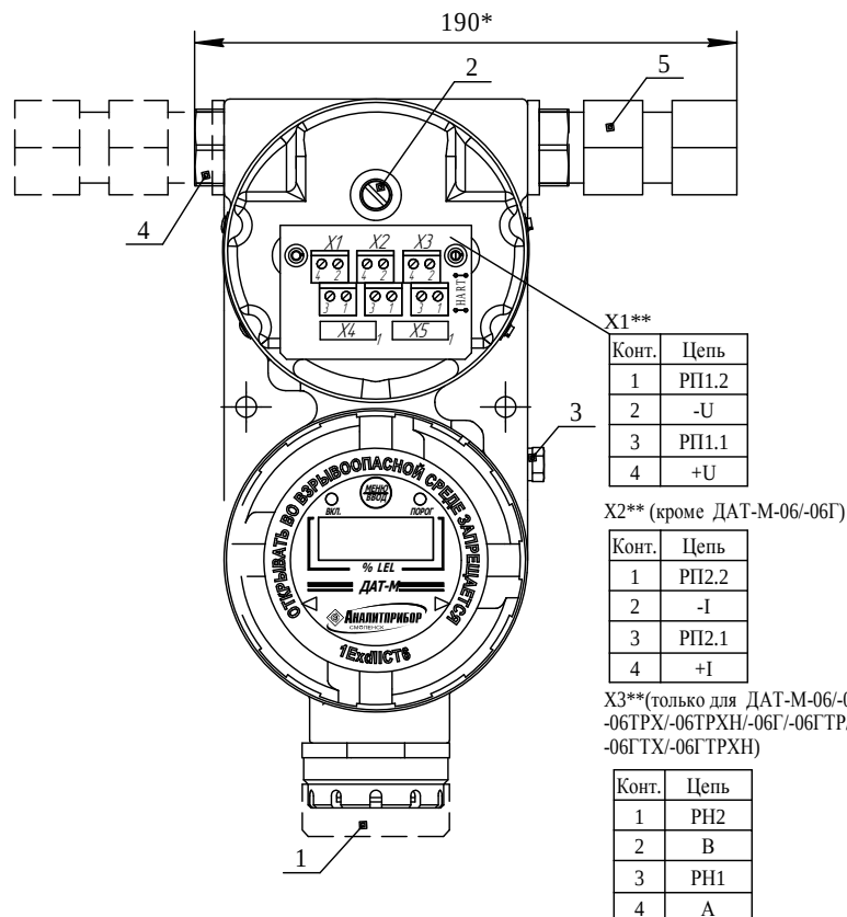
в) сигнализаторы ДАТ-М-05/-06 всех исполнений
