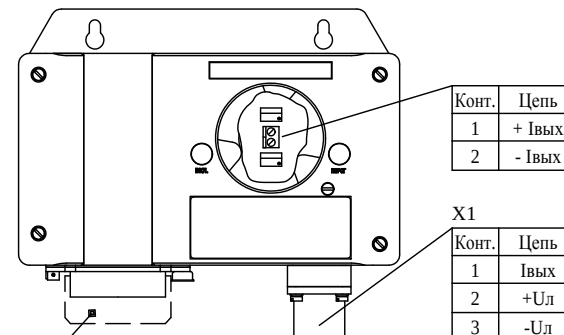
б) сигнализаторы ДАТ-М-02/-03/-04
