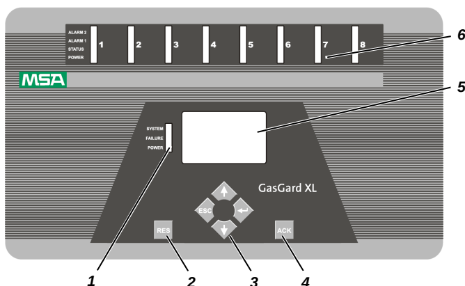
Рис. 3 Панель управления
