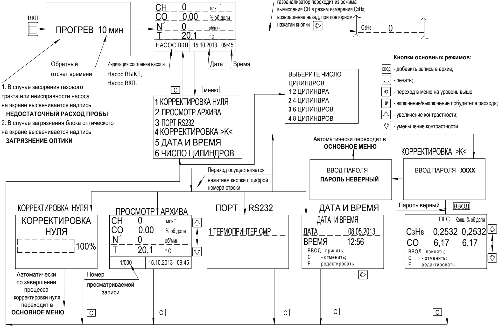
Рисунок 2.16 - Газоанализатор ГИАМ-29М-2. Основное меню
