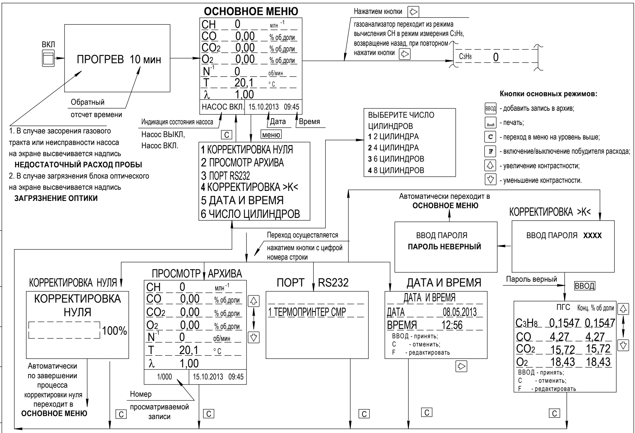
Рисунок 2.1а - Газоанализатор ГИАМ-29М-1. Основное меню
