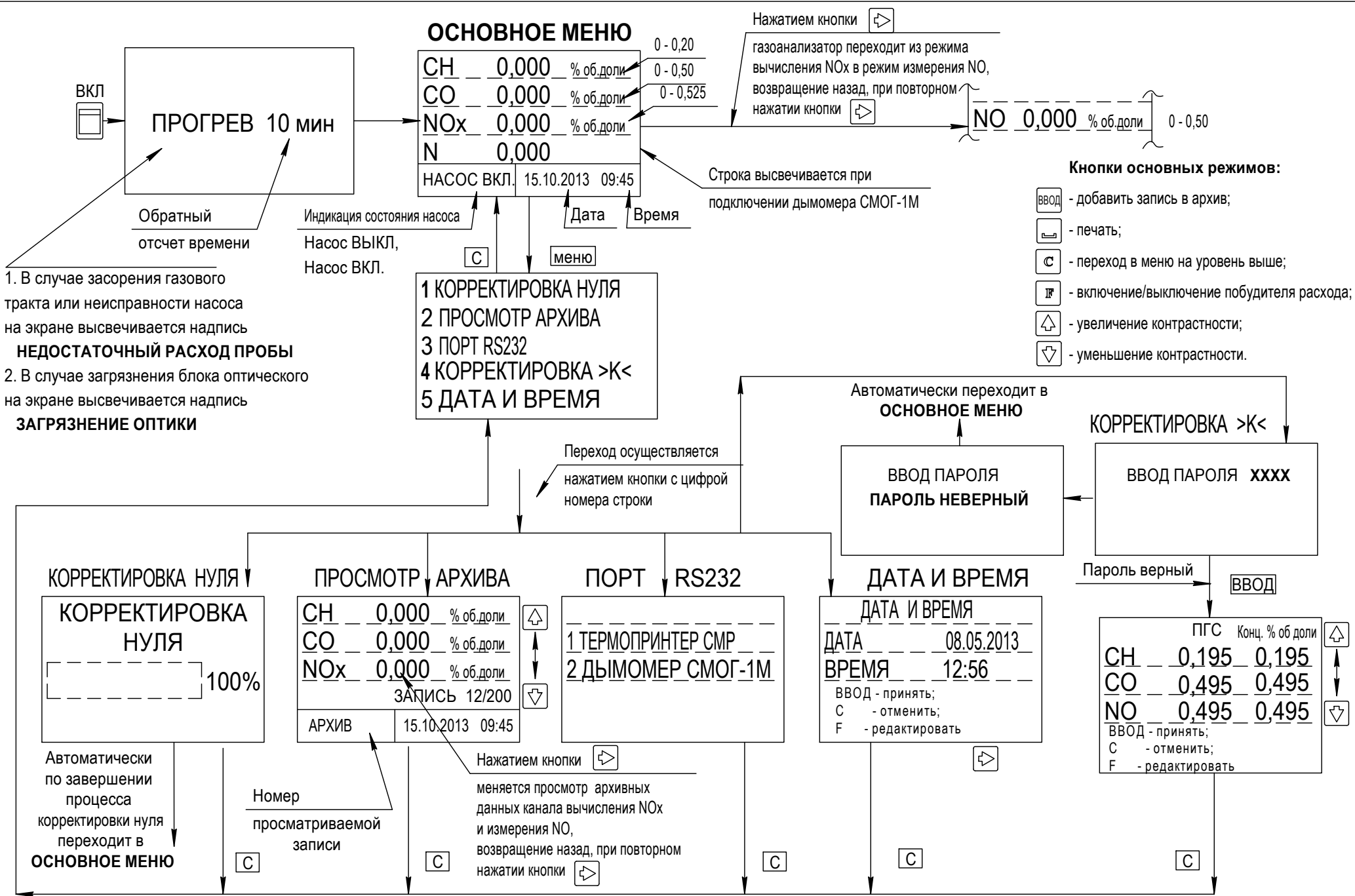
Рисунок 2.1в - Газоанализатор ГИАМ-29М-3. Основное меню
