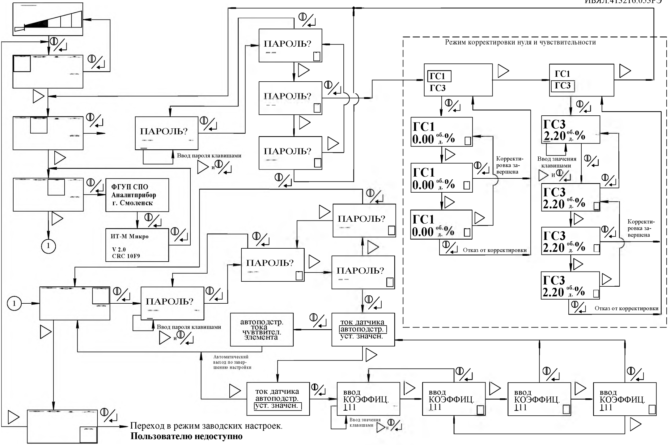
Рисунок Б.1 - Алгоритм режимов работы индикатора
