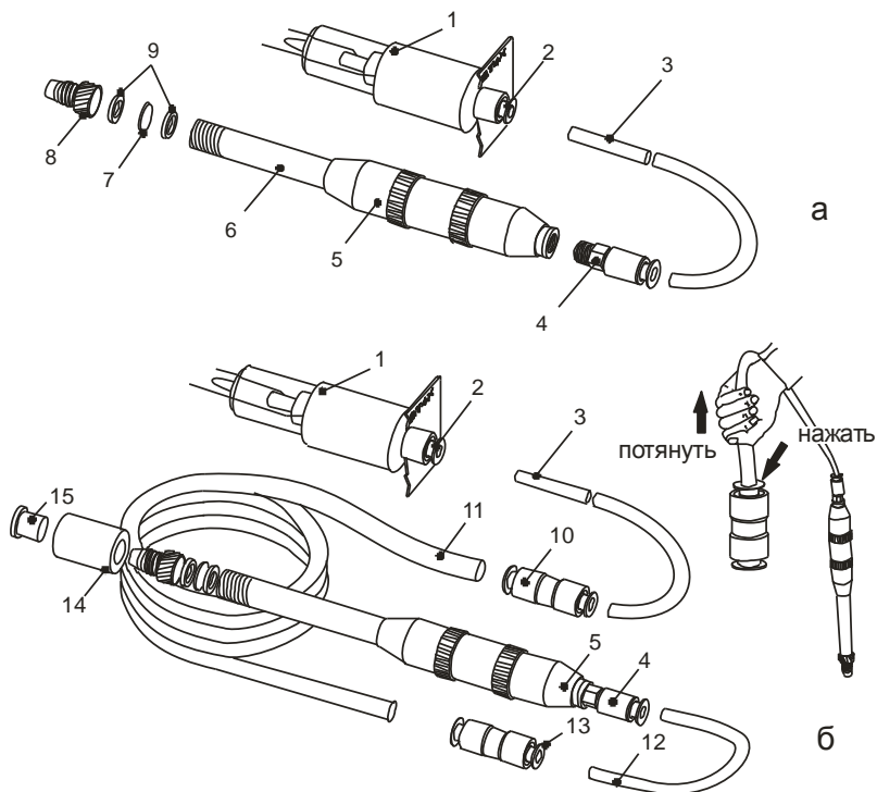
Рис. 4. Схема соединения элементов робоотборника с газоанализатором (а) и элементов удлинителя с газоанализатором (б):
