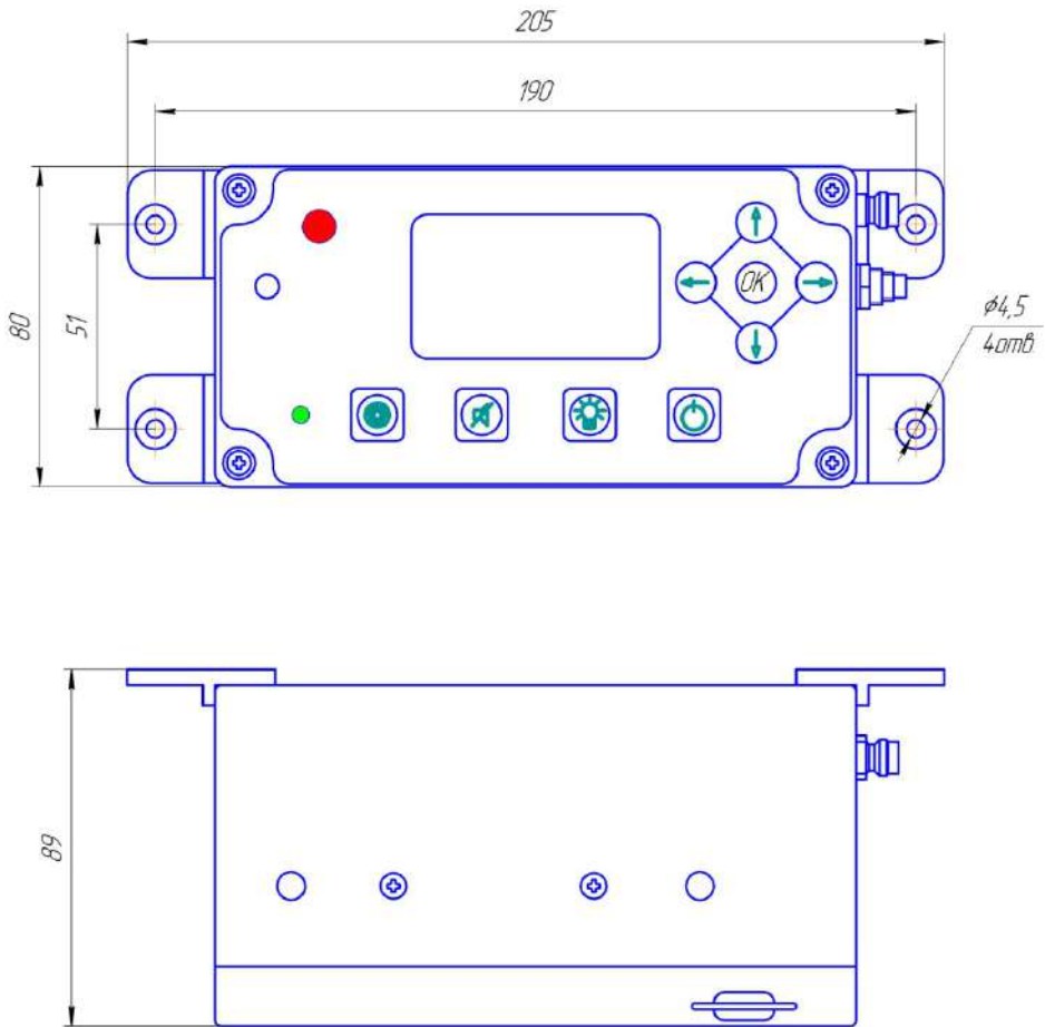
Рисунок 1. Габаритный чертёж
