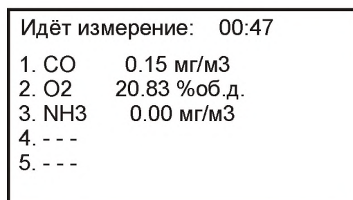
Рисунок 2.10. Вид дисплея газоанализатора в режиме измерения средневзвешенных концентраций
