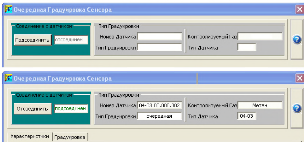
Рисунок Б.8 Программное подсоединение/отсоединение градуировочного блока
