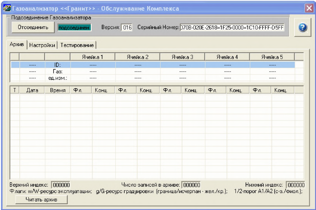
Рисунок Б.2 Страница архивации после подсоединения газоанализатора
