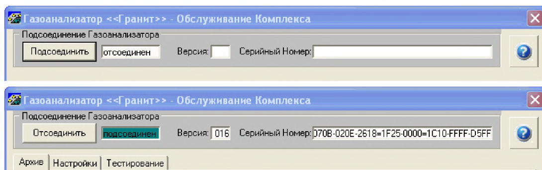
Рисунок Б.1 Программное подключение/отсоединение газоанализатора
