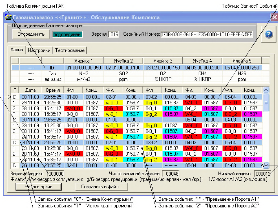
Рисунок Б.4 Пример отображения произошедших событий на странице архив
