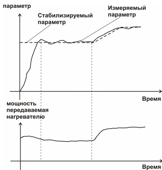
Рисунок 3.11 Стабилизация по ПИД закону
