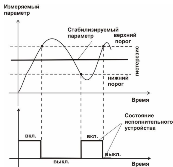
Рисунок 3.10 Стабилизация с гистерезисом
