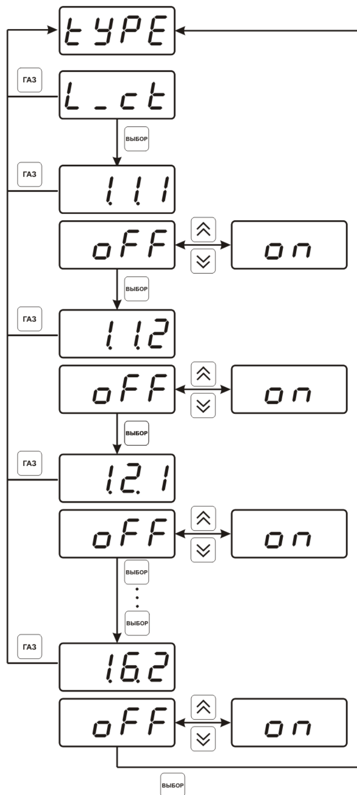
Рисунок 6.19 Настройка логического сигнализатора
