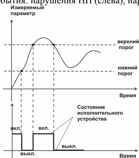
Рисунок 3.9 Функция вида f = НП + ВП
