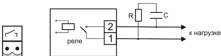
Рисунок 3.6 Подключение нагрузки к выходу управления
