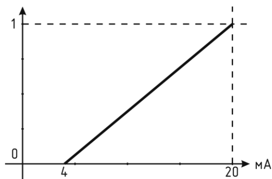
Рисунок 3.12 Линейный выход 4...20 мА с диапазоном 0...1%
