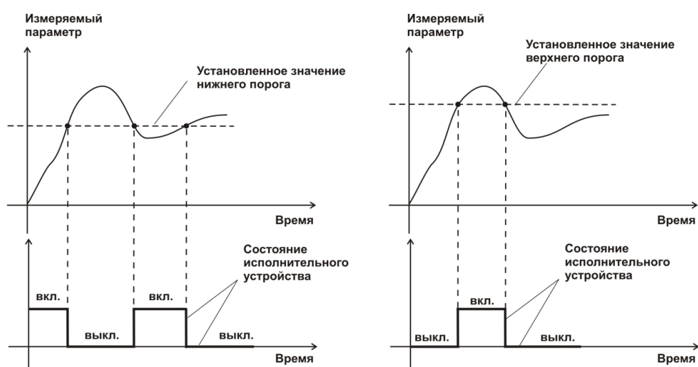
Рисунок 3.8 События: нарушения НП (слева), нарушение ВП (справа)
