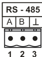
Рисунок 3.5 Вид разъема RS-485
