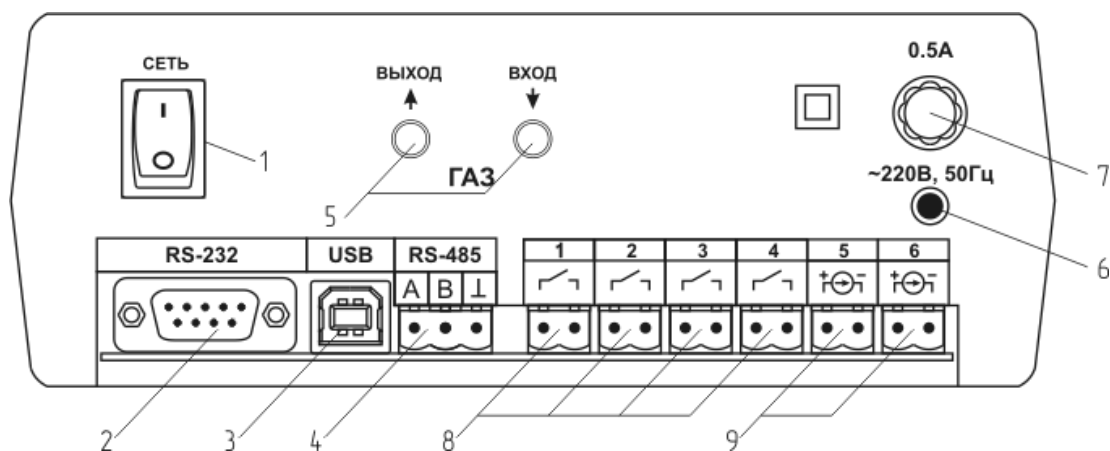
Рисунок 3.2 Задняя панель приборов
