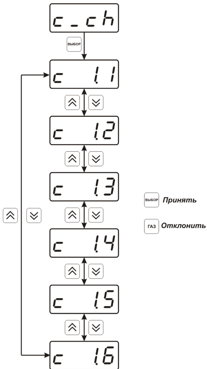
Рисунок 6.15 Настройка входного параметра канала управления (реле)
