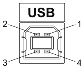
Рисунок 3.4 Разъем USB (розетка «B»)
