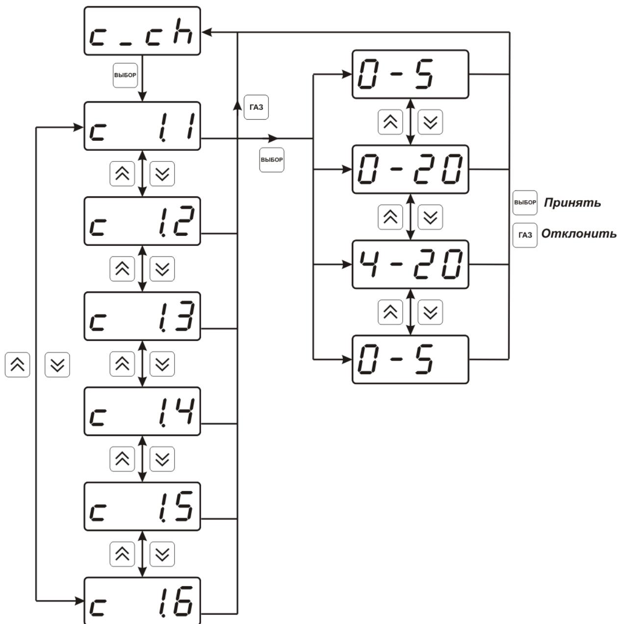
Рисунок 6.16 Настройка входного параметра канала управления (токовый выход)
