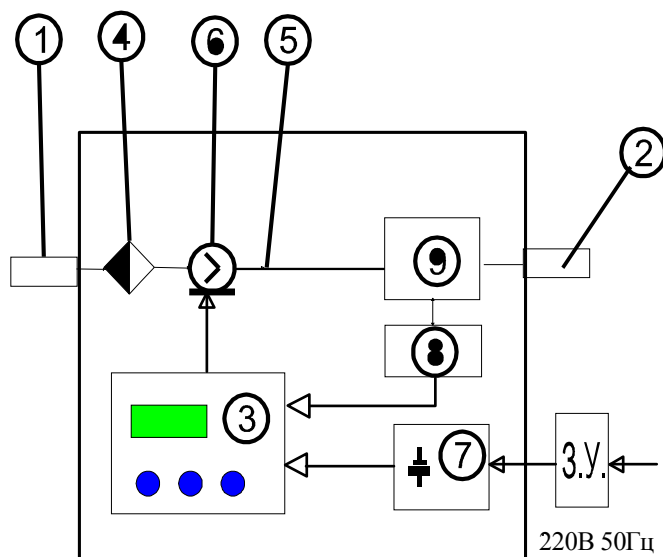
Рис 5.3 Блок-схема газоанализатора
