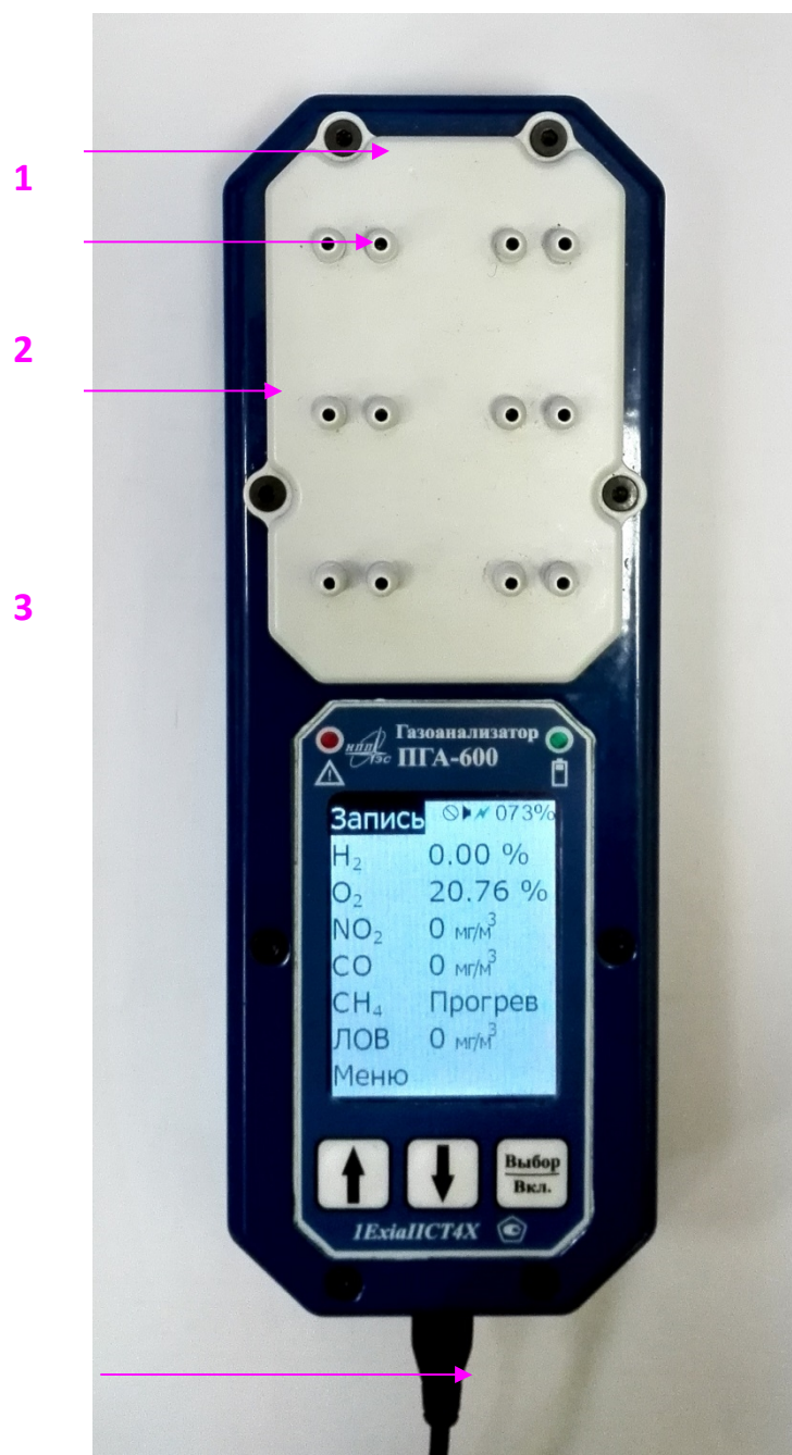
Рисунок А - Общий вид газоанализатора ПГА-600 с установленной калибровочной камерой.
