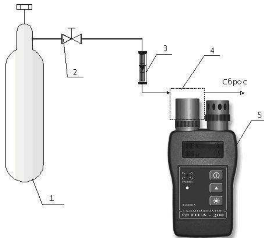
Схема подачи ГСО-ПГС на газоанализаторы ПГА-300
