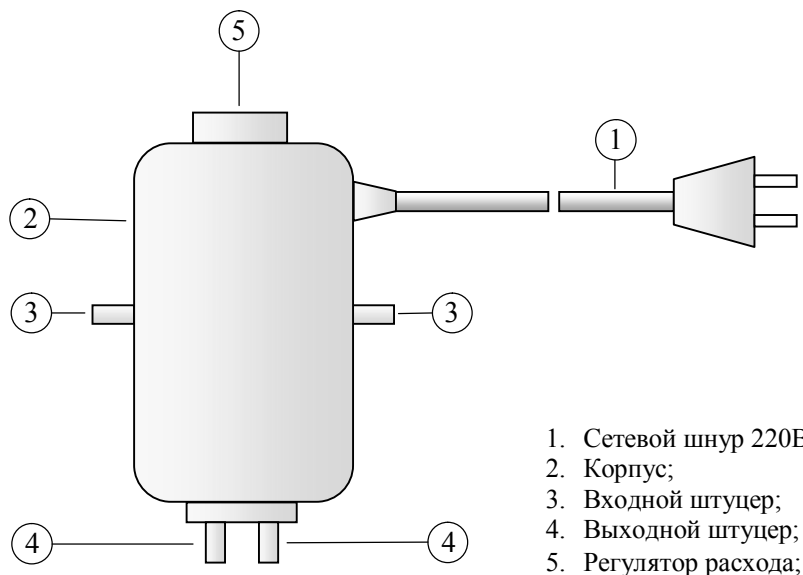
Рис.1. Внешний вид побудителя расхода ПР-2АМ.
