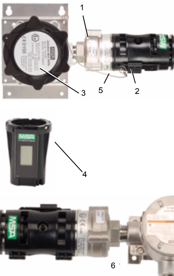
Рис. 1 Общий вид деталей газоанализатора Prima X IR
