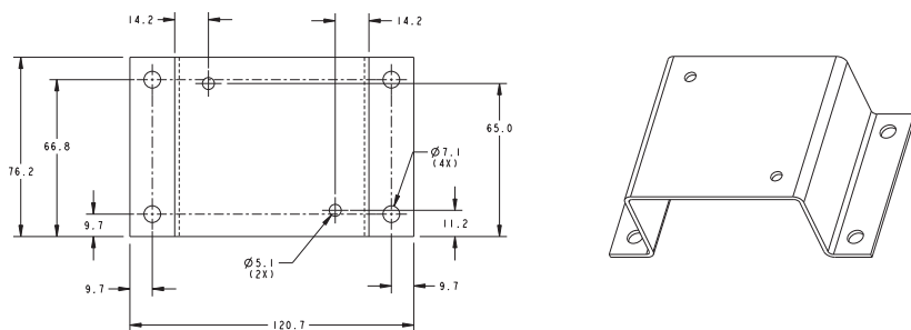
Рис. 6 Монтажный кронштейн для распределительной коробки из нержавеющей стали
