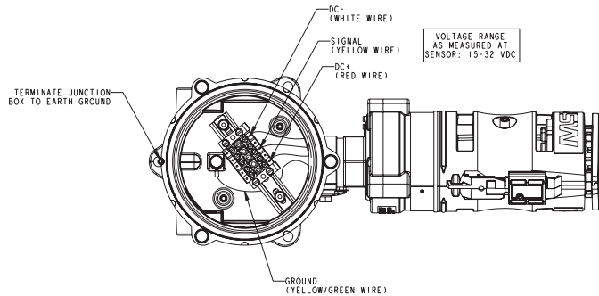
Рис. 7 Схема подключения датчика
