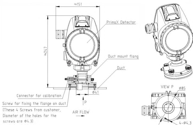
Рис. 26 Монтаж воздуховода
