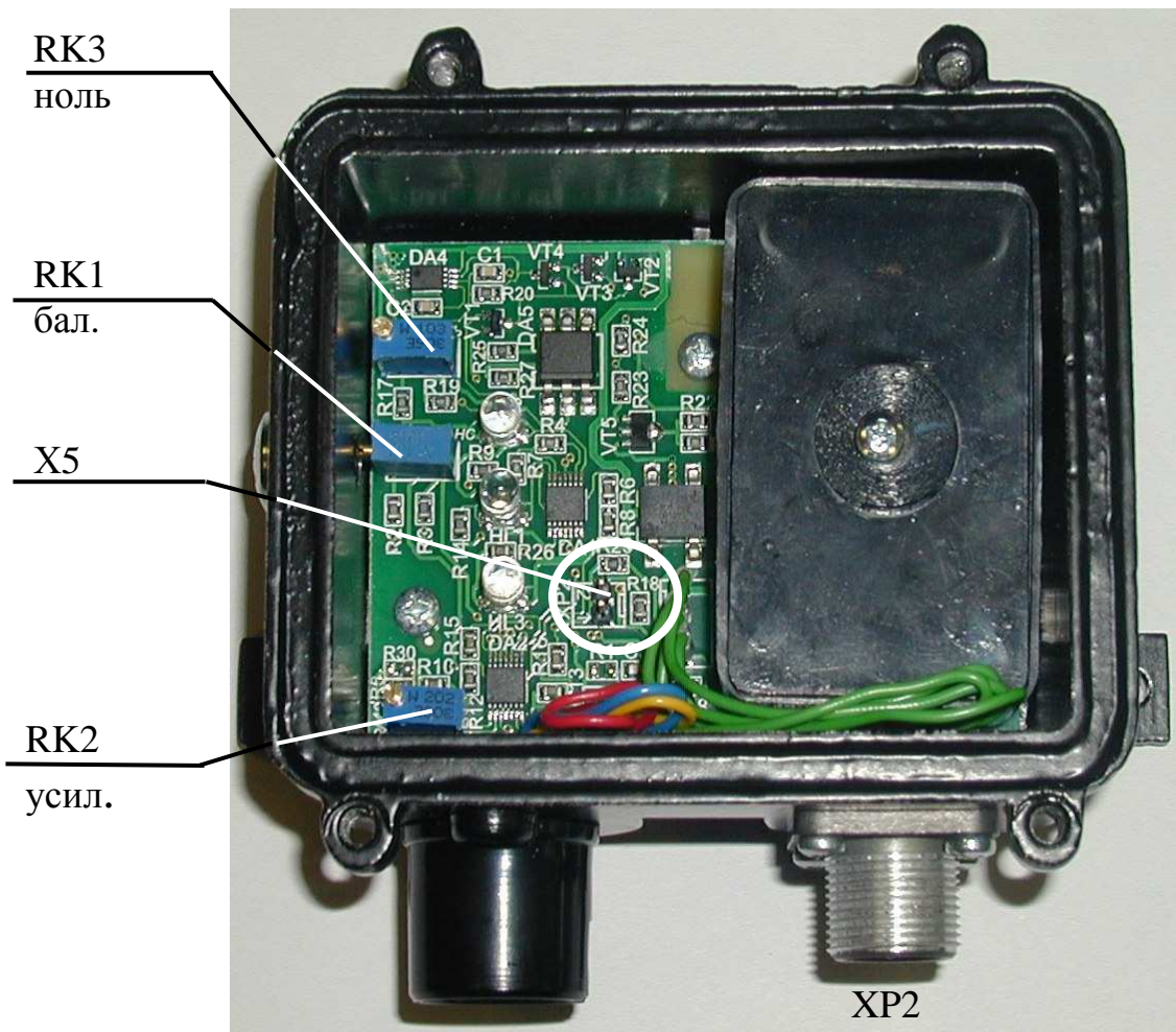
Вид сверху со снятой крышкой
