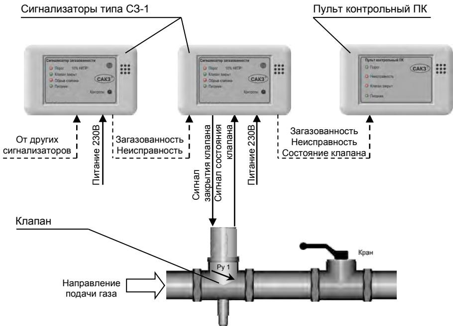
Рисунок 1 – Структурная схема
