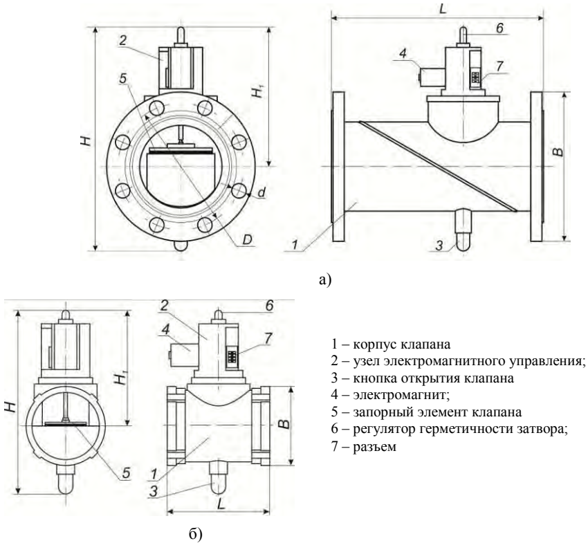
Рисунок 7 – Внешний вид клапана КЗГЭМ-У: а) фланцевый; б) муфтовый
