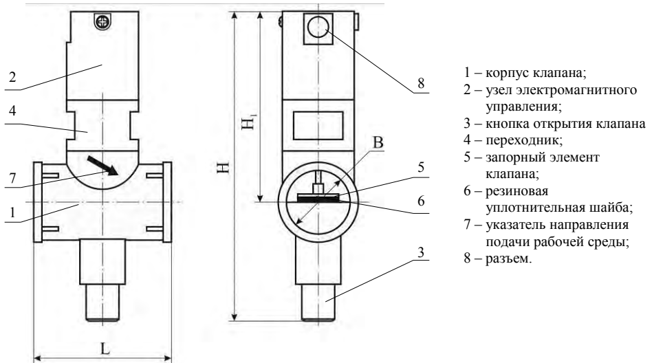
Рисунок 5 – Внешний вид клапана КЗЭУГ.
