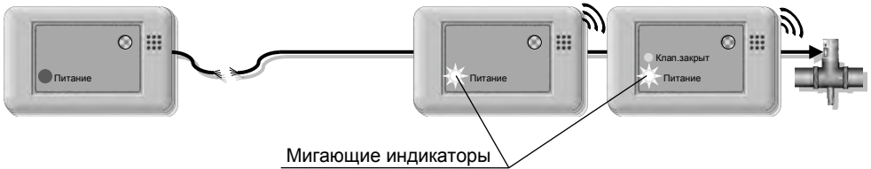
Рисунок 3 – Реакция Системы на обрыв кабеля
