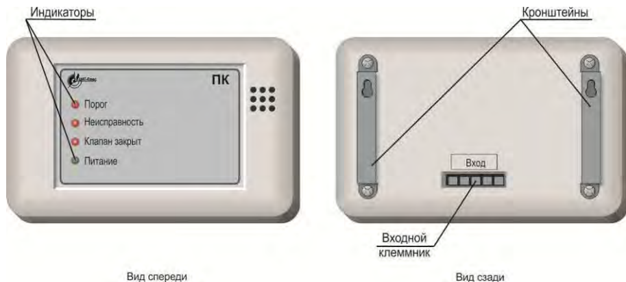
Рисунок 9 – Внешний вид пульта
