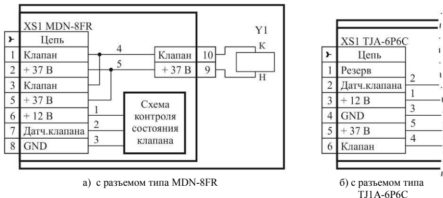
Рисунок 6 – Клапан КЗЭУГ. Схема электрическая принципиальная.
