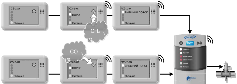
Рисунок 2 – Реакция системы на загазованность.
