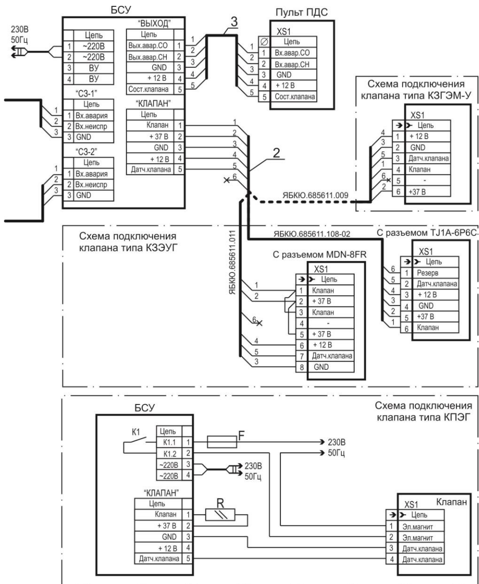
Рисунок Б.1 – САКЗ-МК-2. Схема электрическая соединений (продолжение)
