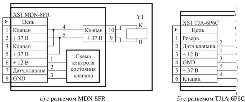
Рисунок 6 – Клапан КЗЭУГ. Схема электрическая принципиальная.
