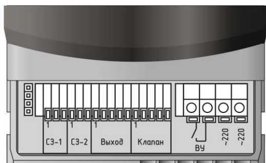
Рисунок 10 – Внешний вид клеммного отсека
