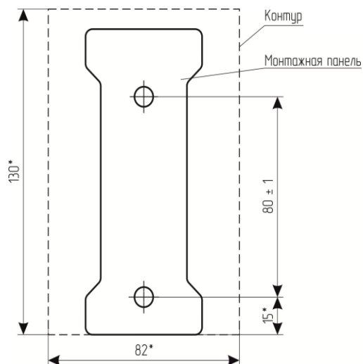
Рисунок В.2 – Разметка крепежных отверстий для БСУ
