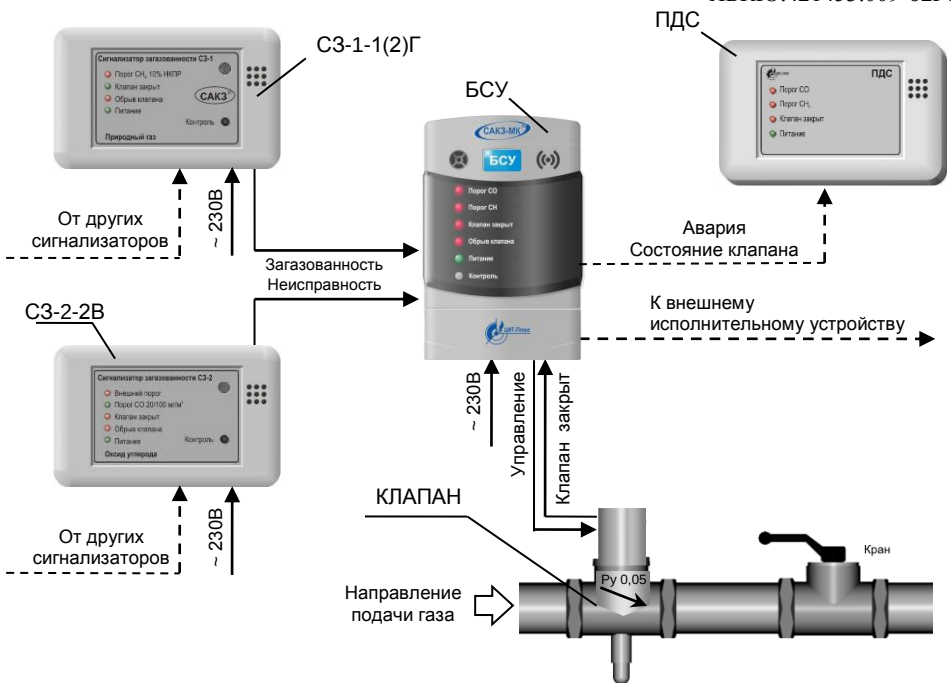
Рисунок 1 - САКЗ-МК-2. Структурная схема
