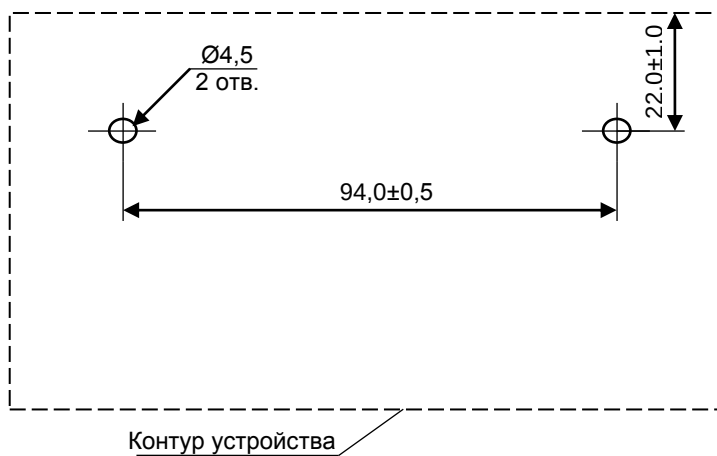
Рисунок В.1 – Разметка крепежных отверстий для сигнализаторов и пульта
