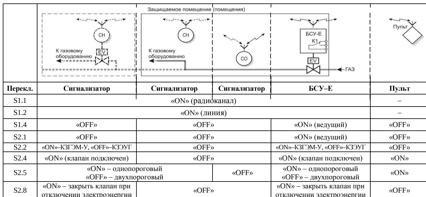
Рисунок 7 – Система с радиоканалом (линия)
