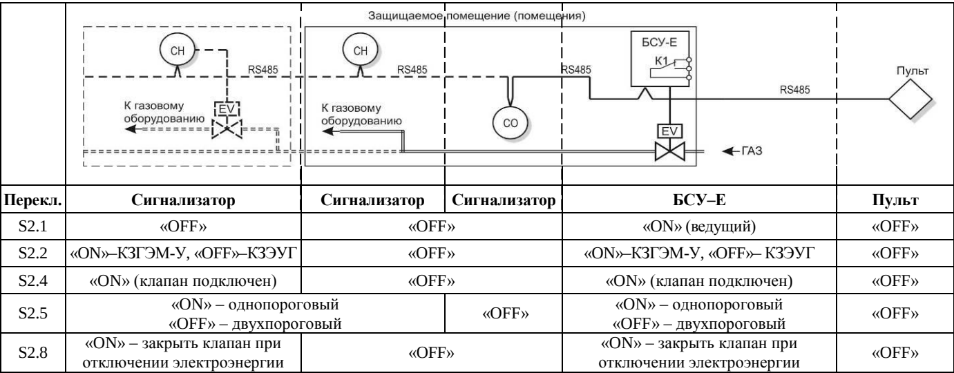
Рисунок 6 – Система с RS485.
