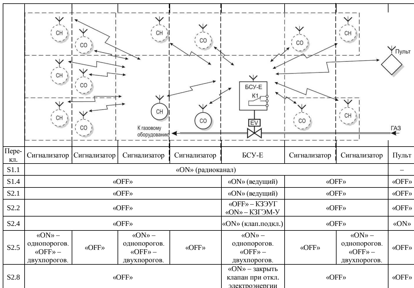
Рисунок 8 – Система с радиоканалом (звезда)
