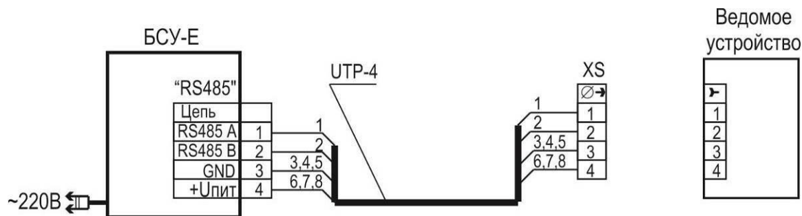
Рисунок Л.1 – Схема соединений для программирования адресов
