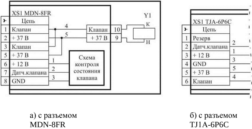
Рисунок 3 – Клапан КЗЭУГ. Схема электрическая принципиальная.
