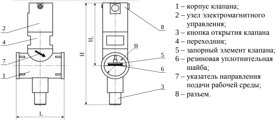
Рисунок 2 – Внешний вид клапана КЗЭУГ.
