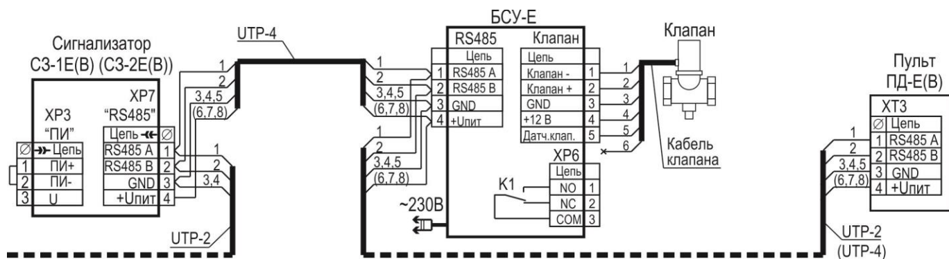
Рисунок Б.1 – Система с RS485.
