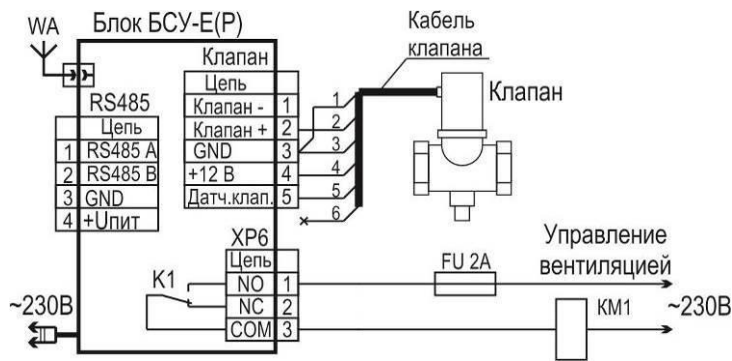
Рисунок Б.5 – Схема управления вентиляцией (S2.5 в положении «ON»)
