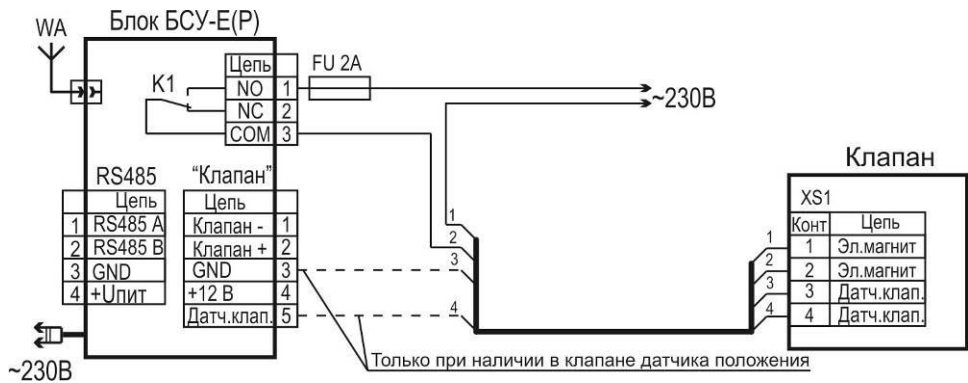
Рисунок Б.4 – Схема подключения клапана типа КПЭГ (S2.5 в положении «OFF»)
