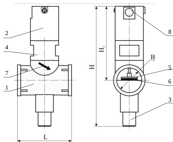
Рисунок 5 – Внешний вид клапана КЗЭУГ.
