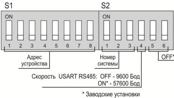
Рисунок 16 – Ретранслятора Р-433. Расположение переключателей.
