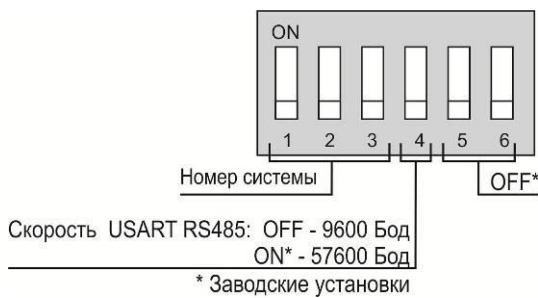
Рисунок 15 – Группа переключателей «Конфигурация»
