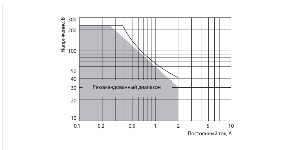
Рис.б. Допустимая мощность коммутации силовых реле
