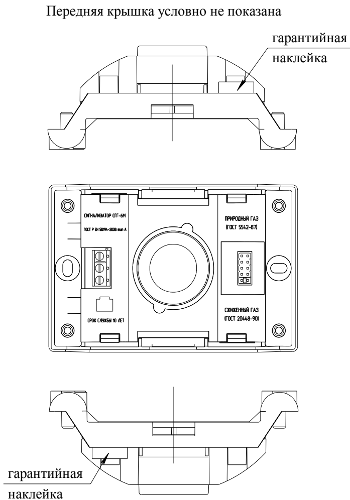
Рисунок 2 - Схема пломбировки сигнализатора от несанкционированного доступа и обозначение мест для нанесения гарантийных наклеек
