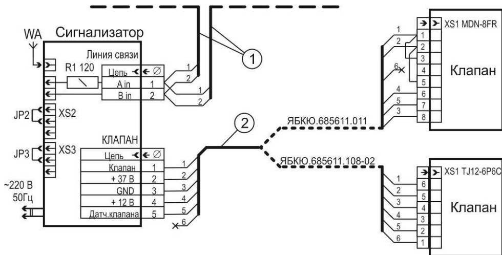
а) с клапаном КЗЭУГ
