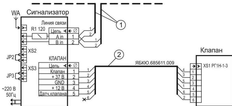
б) с клапаном КЗГЭМ-У
