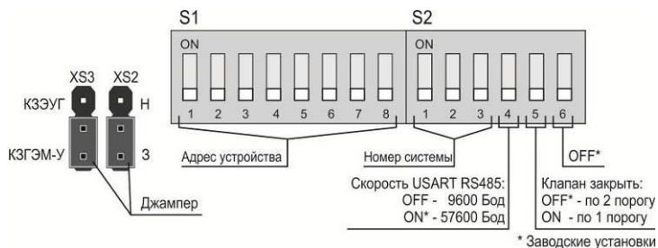
Рисунок 2 – Назначение переключателей и переключек сигнализатора.
