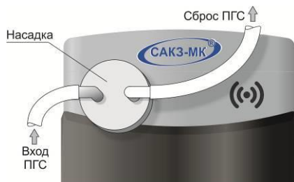
Рисунок Д.2 – Установка насадки для подачи ПГС
