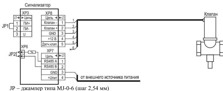
Рисунок В.3 – Схема подключения сигнализатора СЗ-2ЕВ
