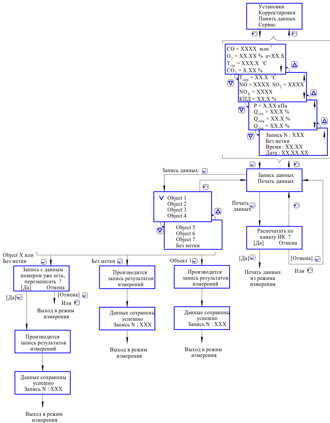
Рисунок 2.11 – Схема режимов работы газоанализаторов при записи и печати
