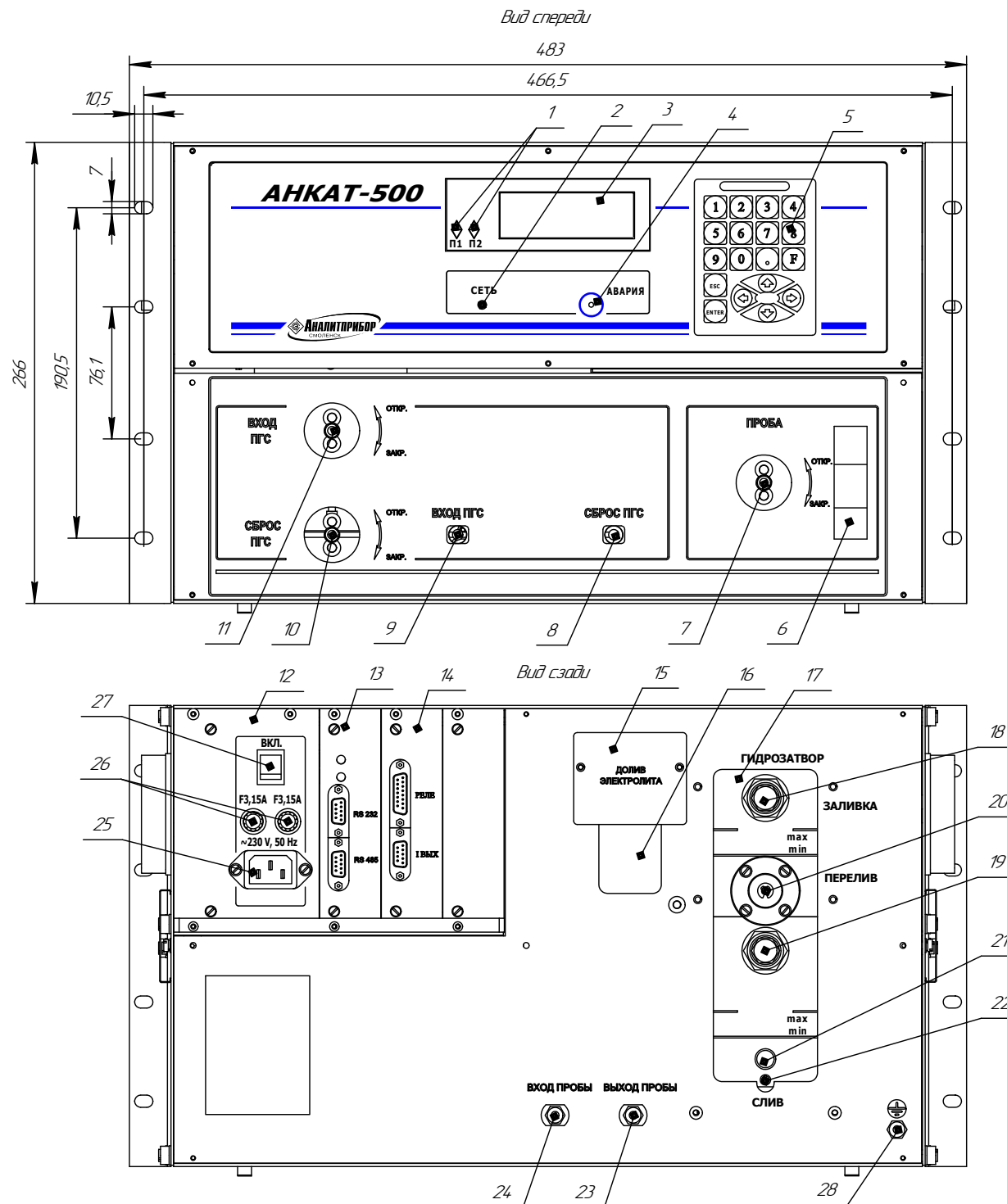
Рисунок 11 – Газоанализаторы АНКAT-500. Внешний вид.
