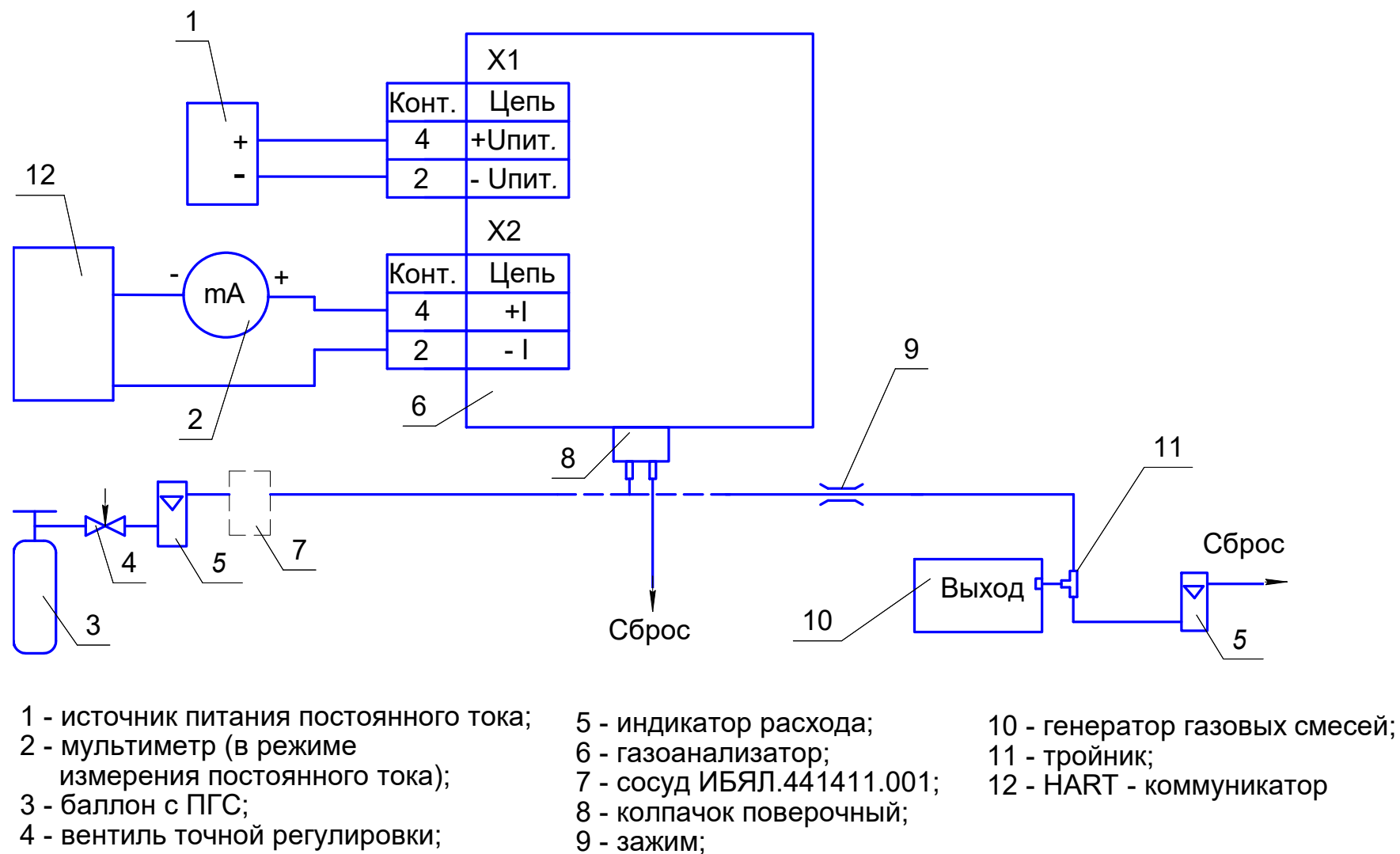
Рисунок К.2 – Схема проверки по ПГС газоанализаторов ДАХ-М-05Х, ДАХ-М-05ХН
