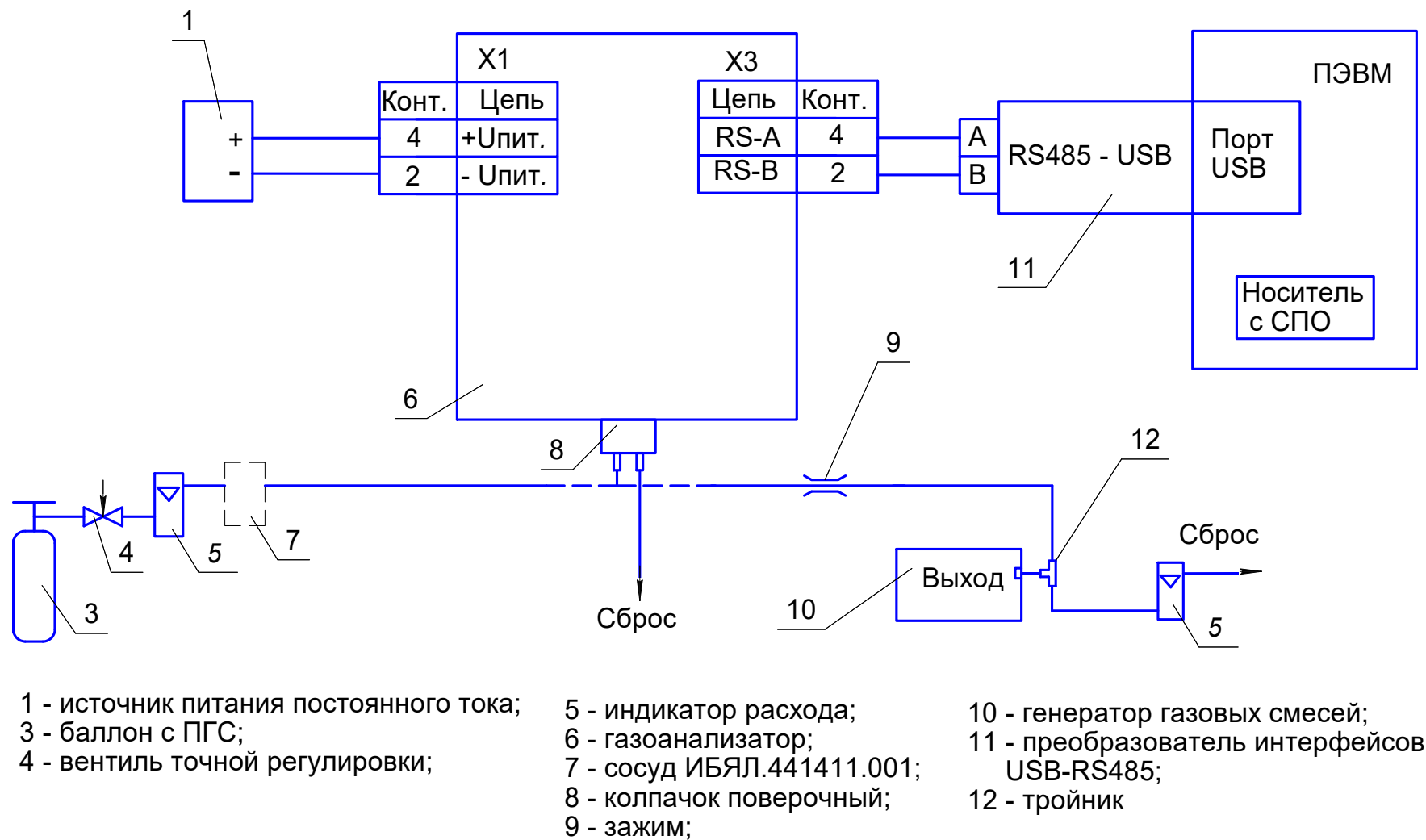
Рисунок К.3 – Схема проверки по ПГС газоанализаторов ДАХ-М-06
