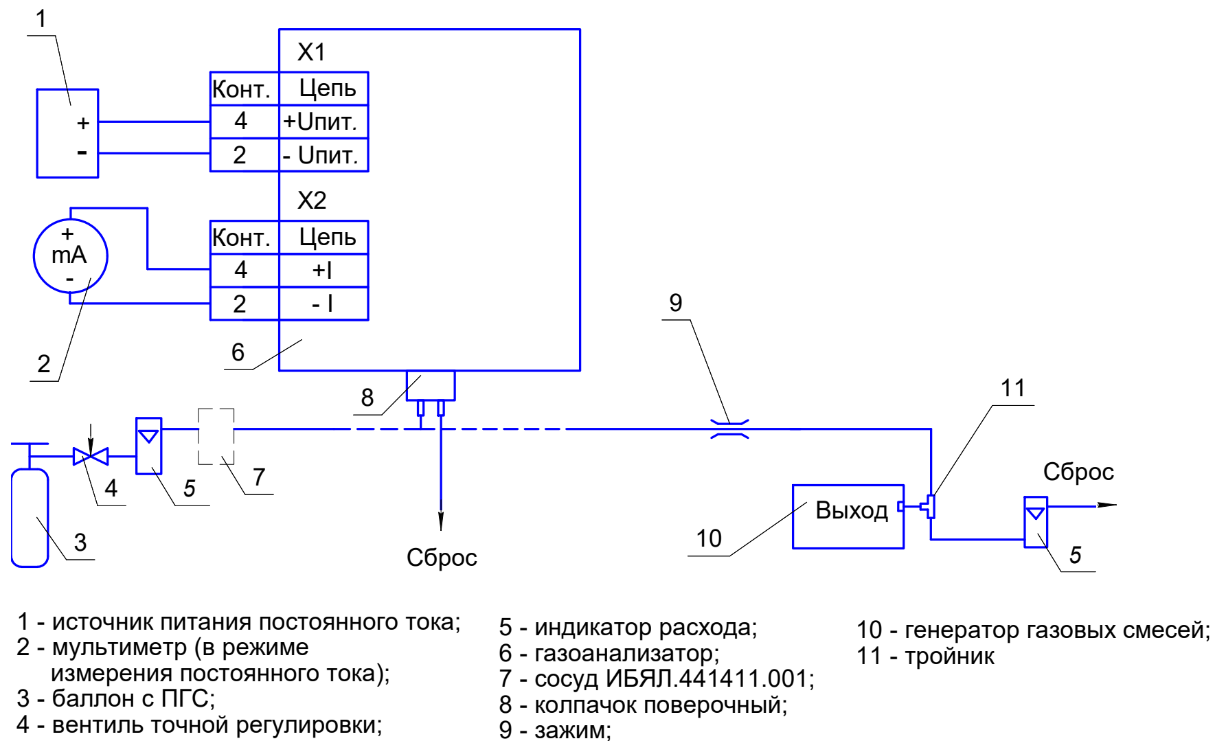
Рисунок К.1 – Схема проверки по ПГС газоанализаторов ДАХ-М-05
