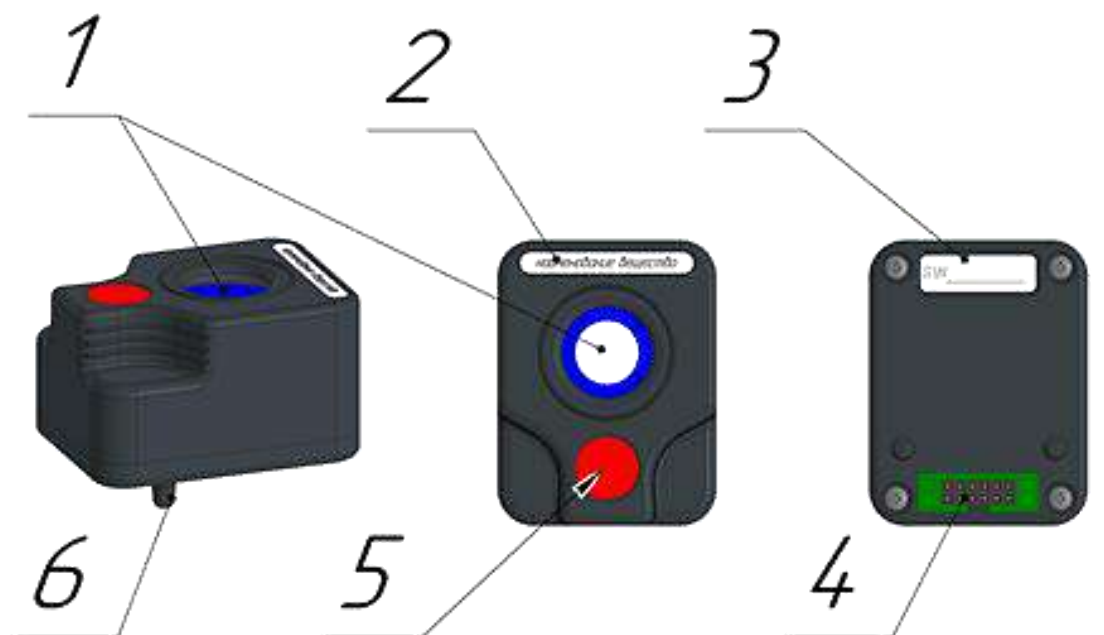
Рисунок 7.2 - Общий вид датчиков «ЭКОЛАБ Плюс»
