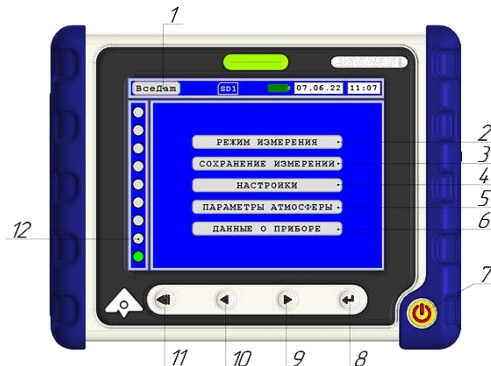
Рисунок 9.6 – Основное меню
