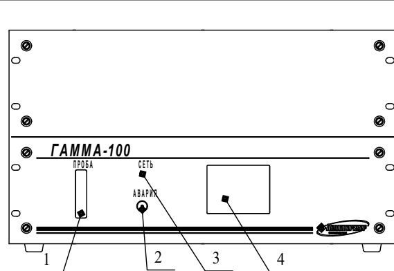
а) газоанализаторы ГАММА-100 (три измерительных канала)
