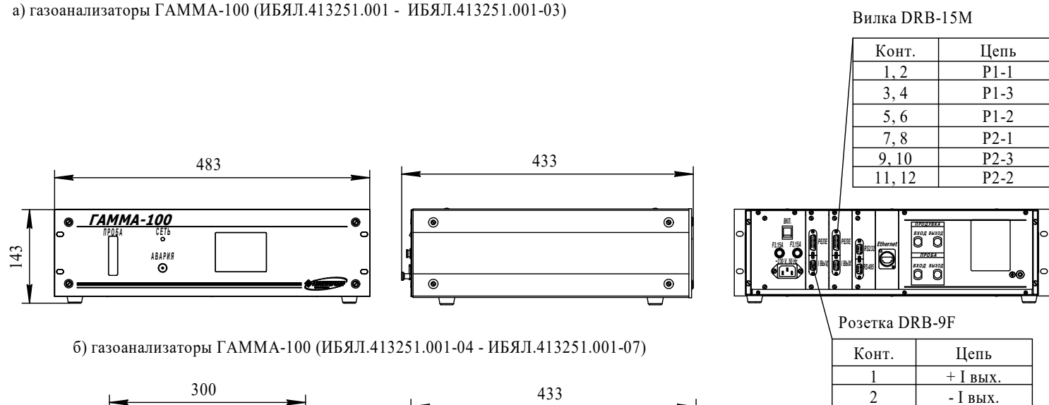
а) газоанализаторы ГАММА-100 (ИБЯЛ.413251.001 - ИБЯЛ.413251.001-03)
