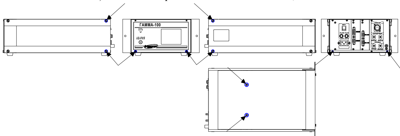
б) газоанализаторы ИБЯЛ.413251.001-04...-07;
