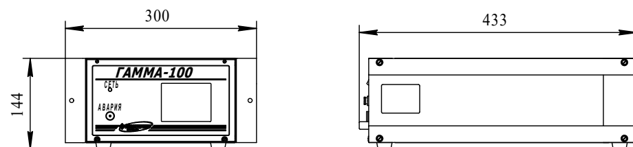
б) газоанализаторы ГАММА-100 (ИБЯЛ.413251.001-04 - ИБЯЛ.413251.001-07)
