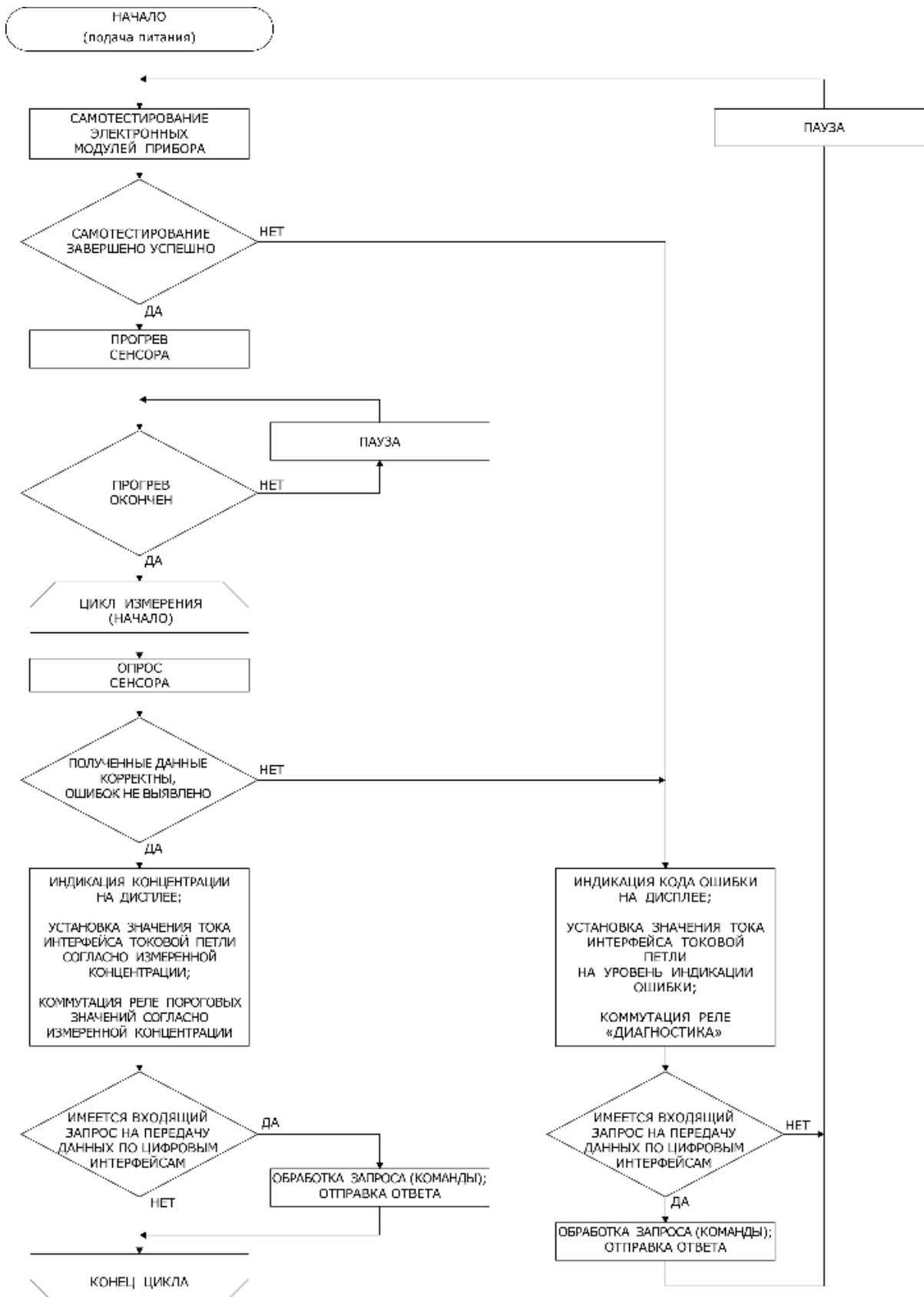
Рисунок 14 – Алгоритм функционирования ИГМ-12М
