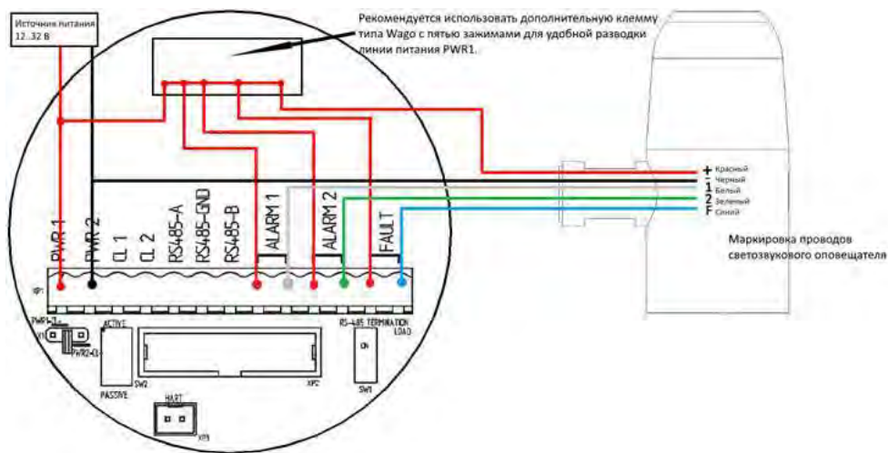
Рисунок 22 – Схема подключения светозвукового сигнализатора ЭМИ-С3 к ИГМ-12М, изготовленным до апреля 2023г.
