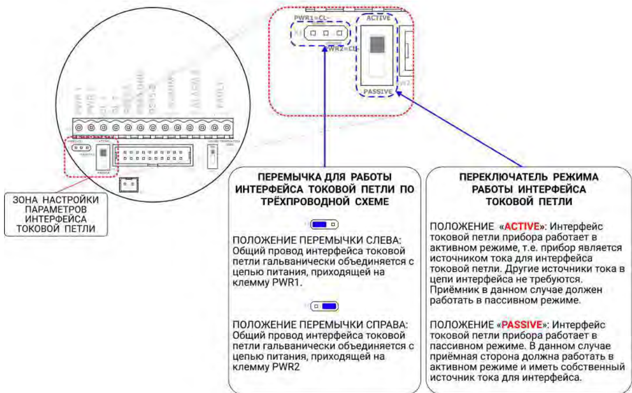
Рисунок 25 – Настройка параметров интерфейса токовой петли для ИГМ-12М, изготовленных до апреля 2023г.
