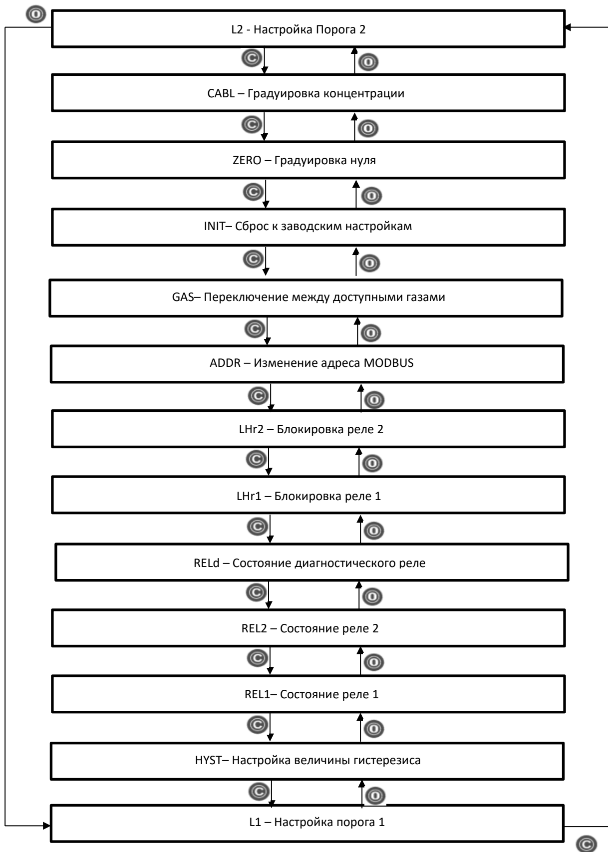
Рисунок К.2.2 – Структура меню
