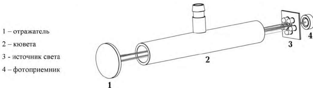
Рис.1. Оптическая схема дымомера
