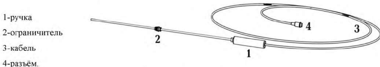
Рис 6. Датчик температуры масла
