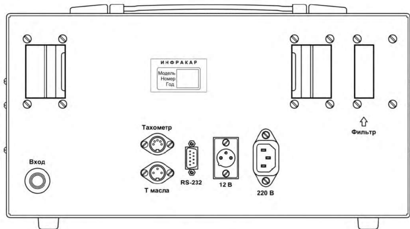
Рис 5а. Вид сзади.
