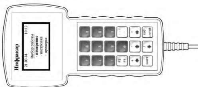
Рис 3. Пульт управления. Вид спереди.
