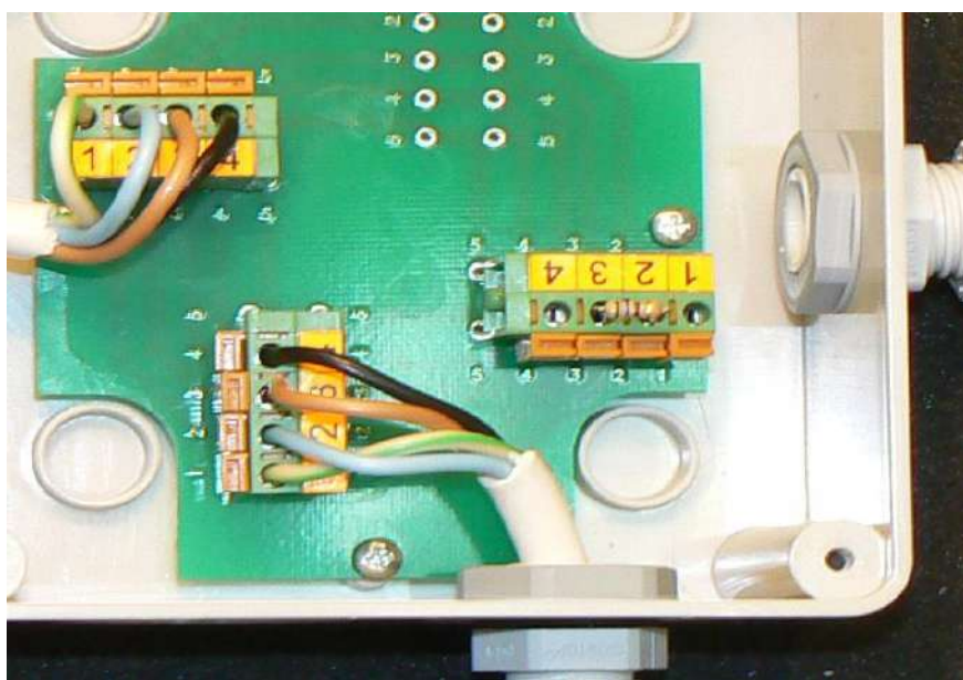
Рис.Д.5. Установка нагрузочного резистора в монтажном комплекте МКУ
