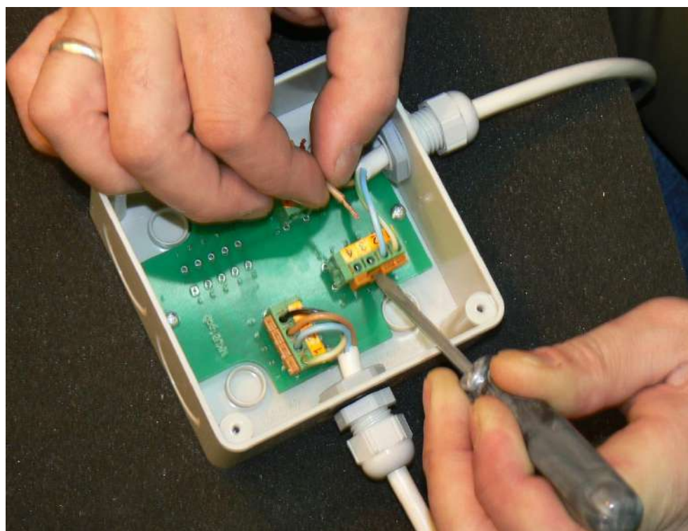
Рис.Д.7. Монтаж кабеля – этап 2.
