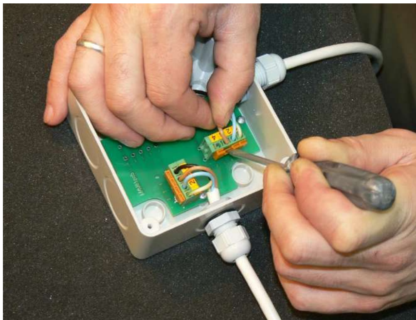
Рис.Д.6. Монтаж кабеля – этап 1.
