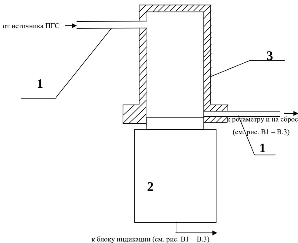
Рис. 3.1. Подача ПГС в адаптер при проверках
