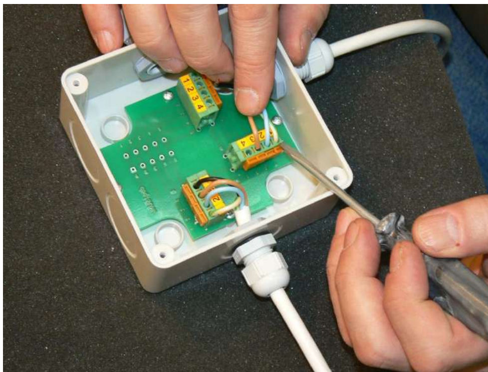
Рис.Д.8 Монтаж кабеля – этап 3.
