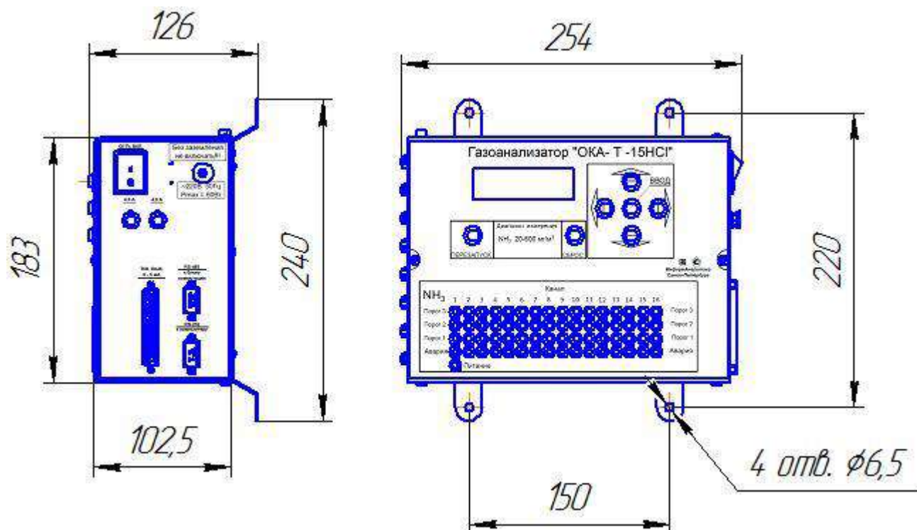
Рис.Е.1. Блок индикации «ОКА-92МТ» исполнение И21.
