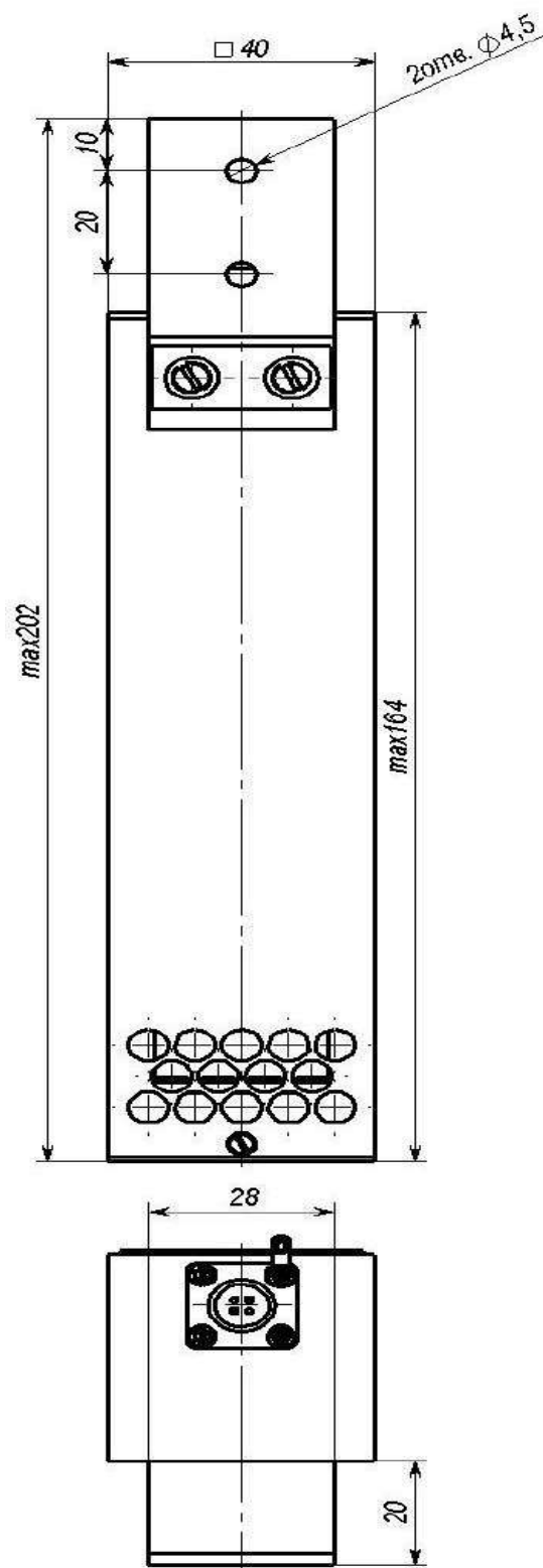
Рис.Е.4. Блок сенсоров (взрывозащищенный).
