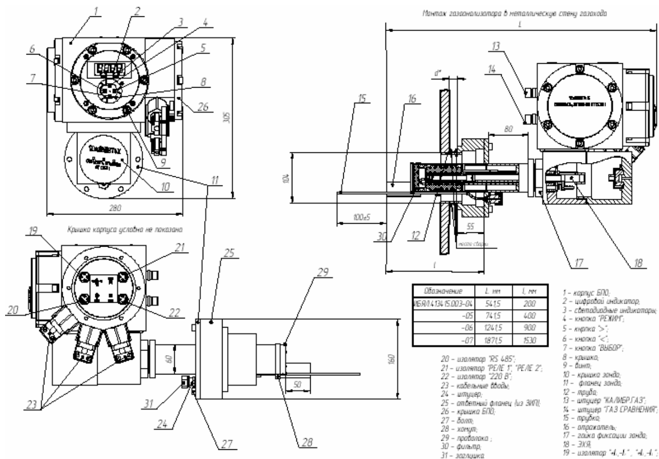
Рисунок 1.1 - Внешний вид газоанализатора АКВТ-02 с разметкой для монтажа
