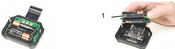
Рис. 13 Замена батареи
