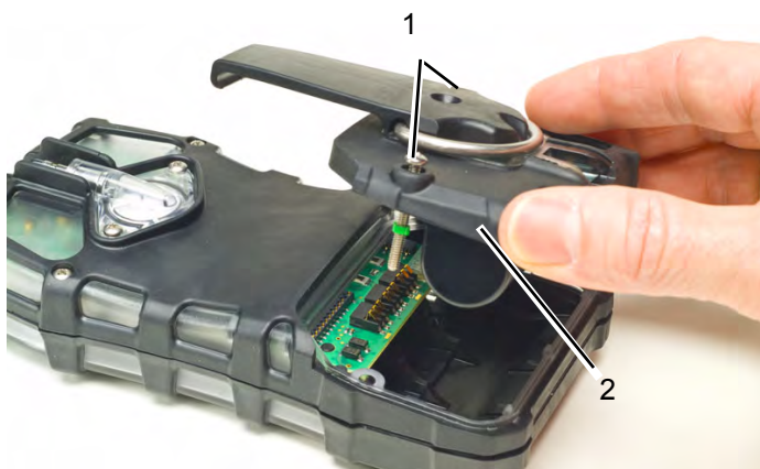
Рис. 12 Замена батареи
